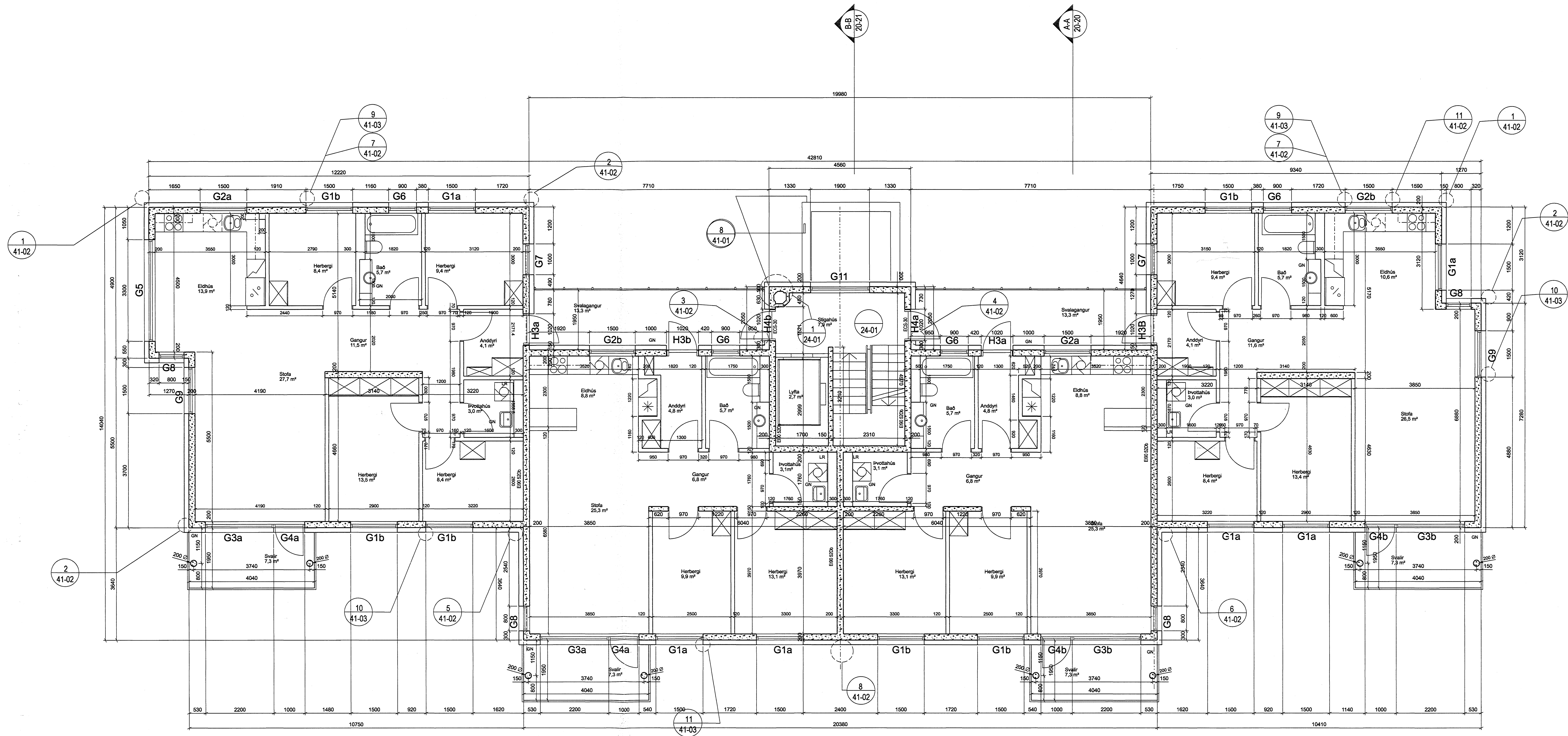
GRUNNMYND 1:50 2-5 hæð
