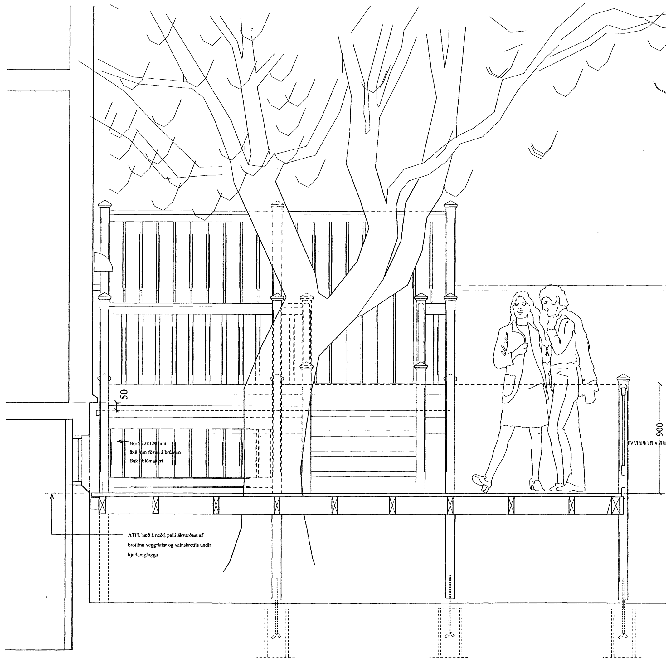
Þversneiðing B-B
