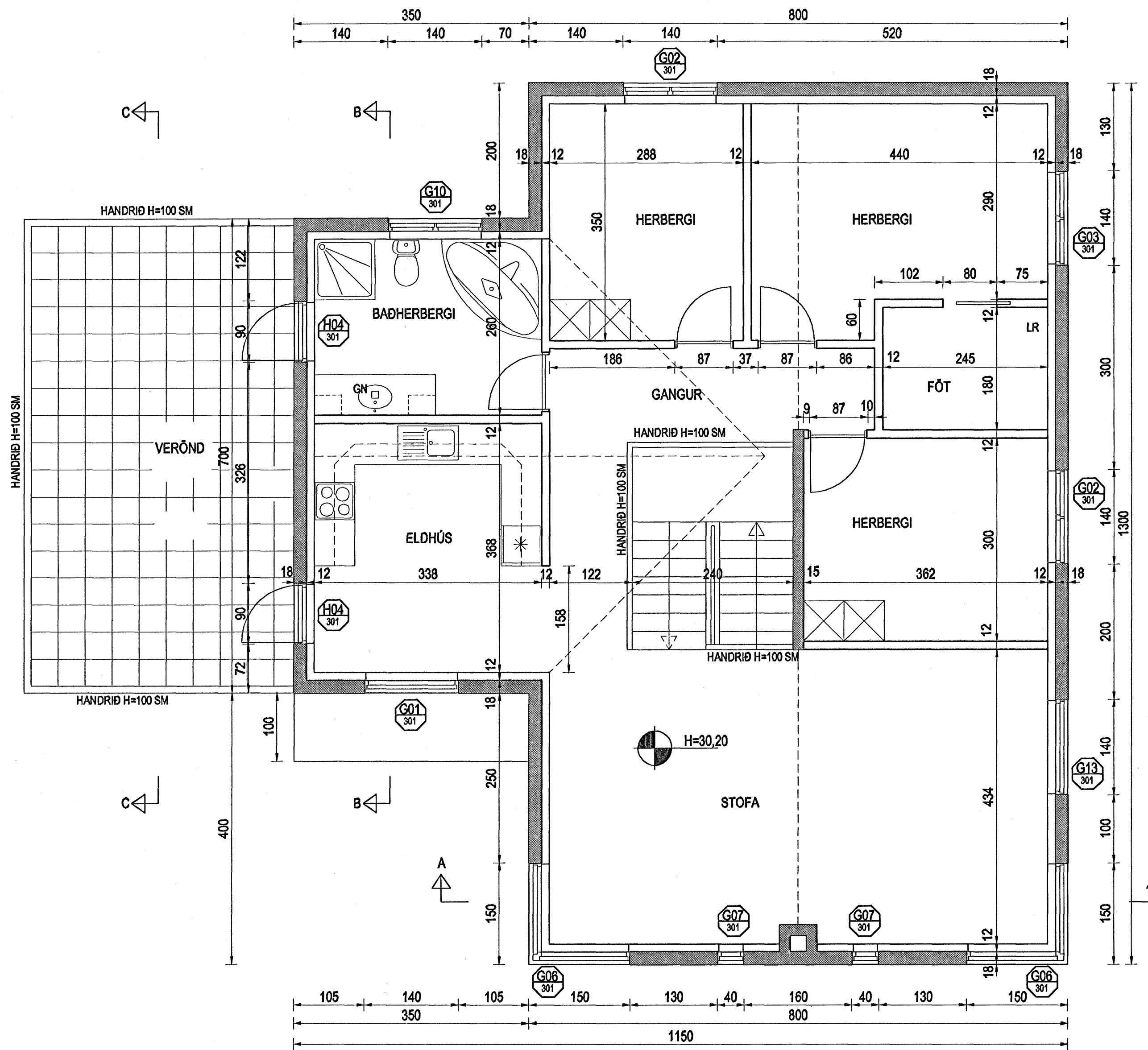
GRUNNMYND EFRI HÆÐAR MKV. 1:50
