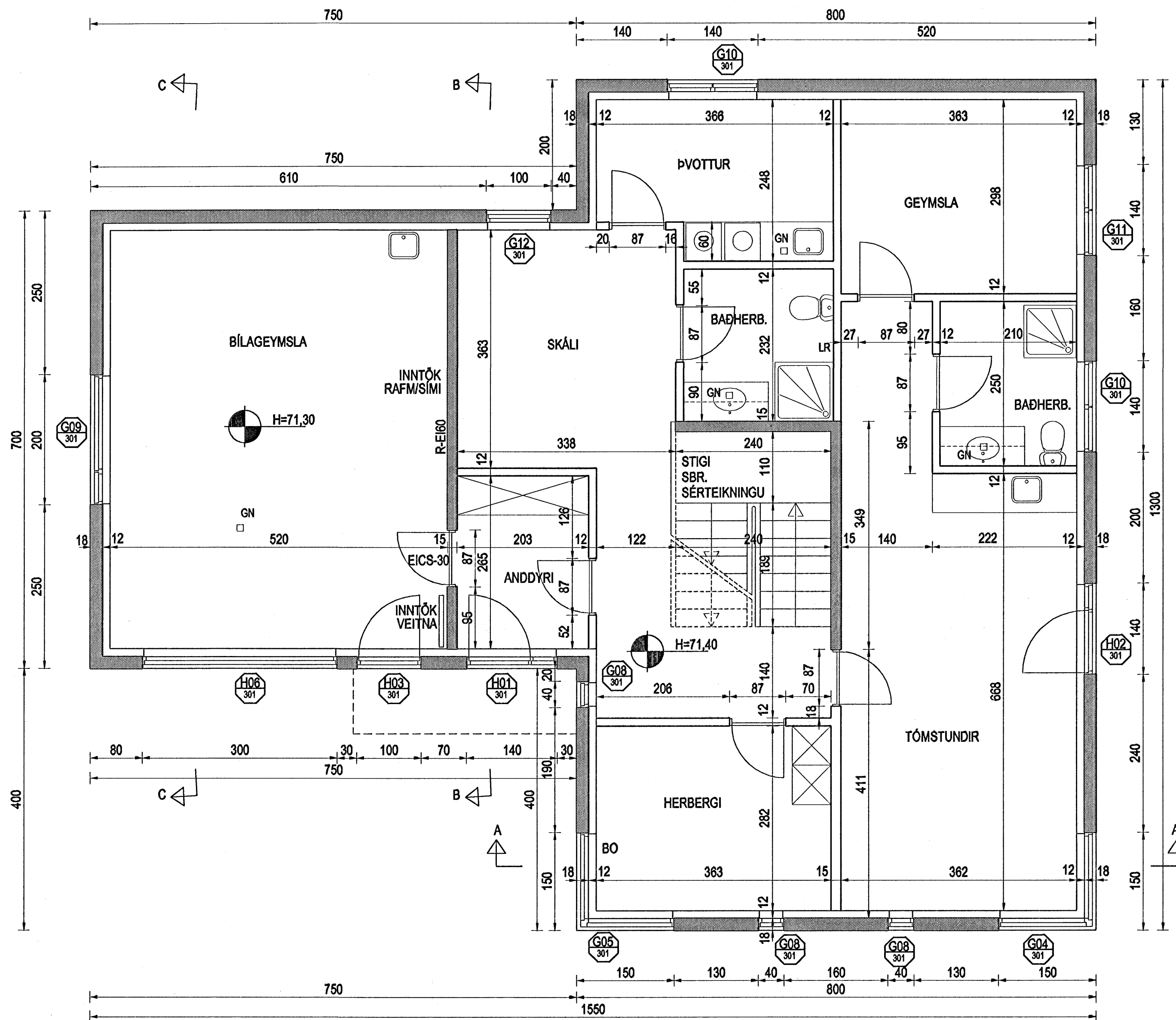
GRUNNMYND NEDRI HÆÐAR MKV. 1:50
