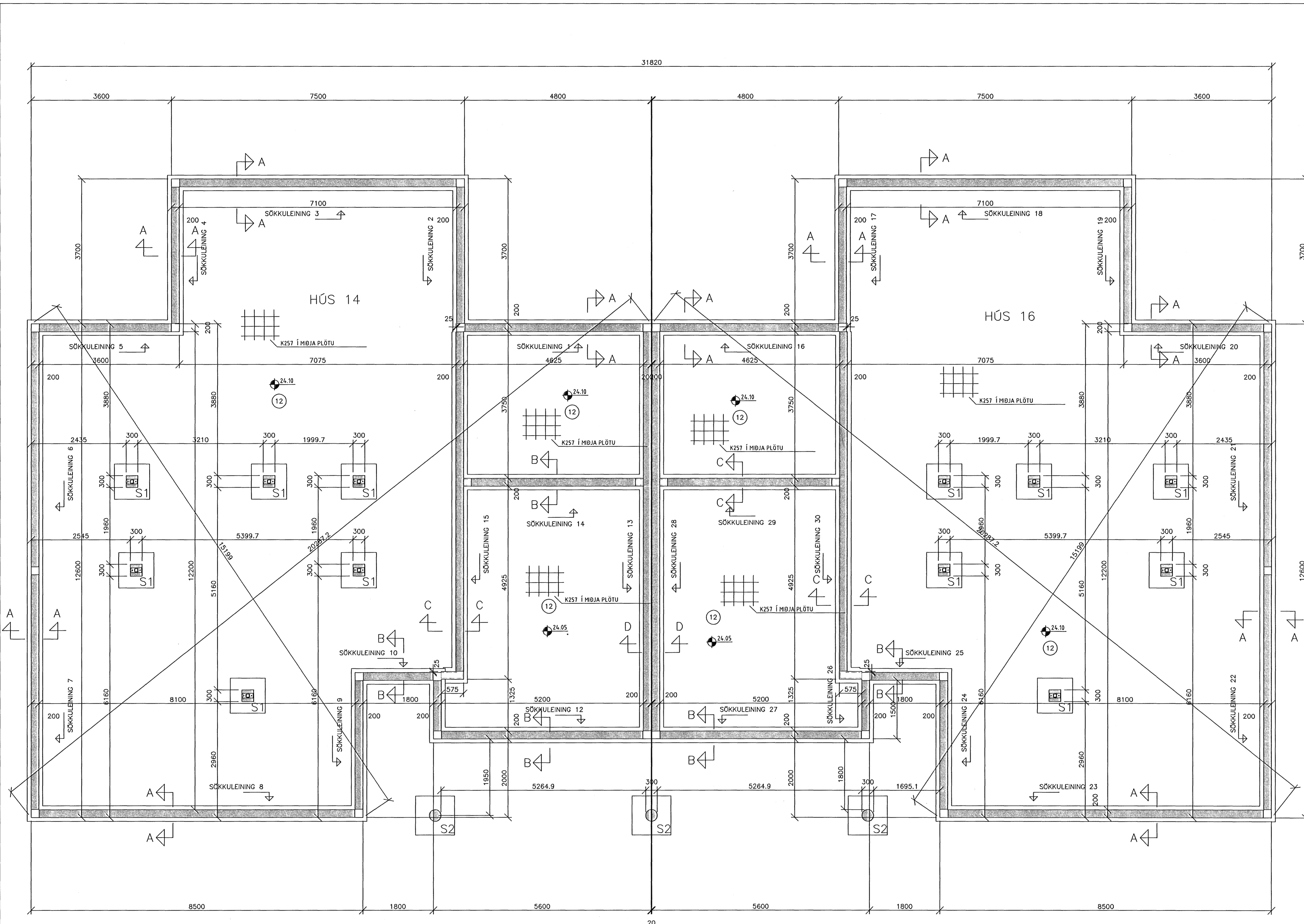
GRUNNMYND SÖKKLA 1:50
