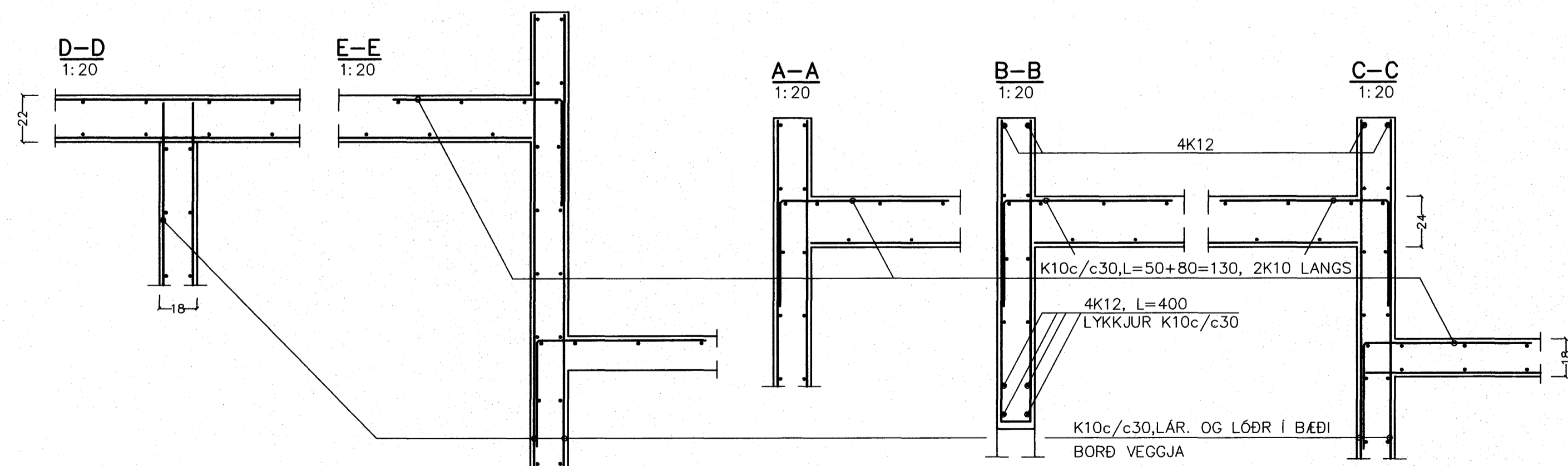
LÁR. SNIÐ Í ÚTHORN VEGGJA F 1:20
