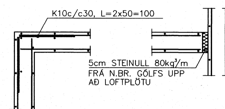
LÁR. SNIÐ Í ÚTHORN VEGGJA F 1:20
