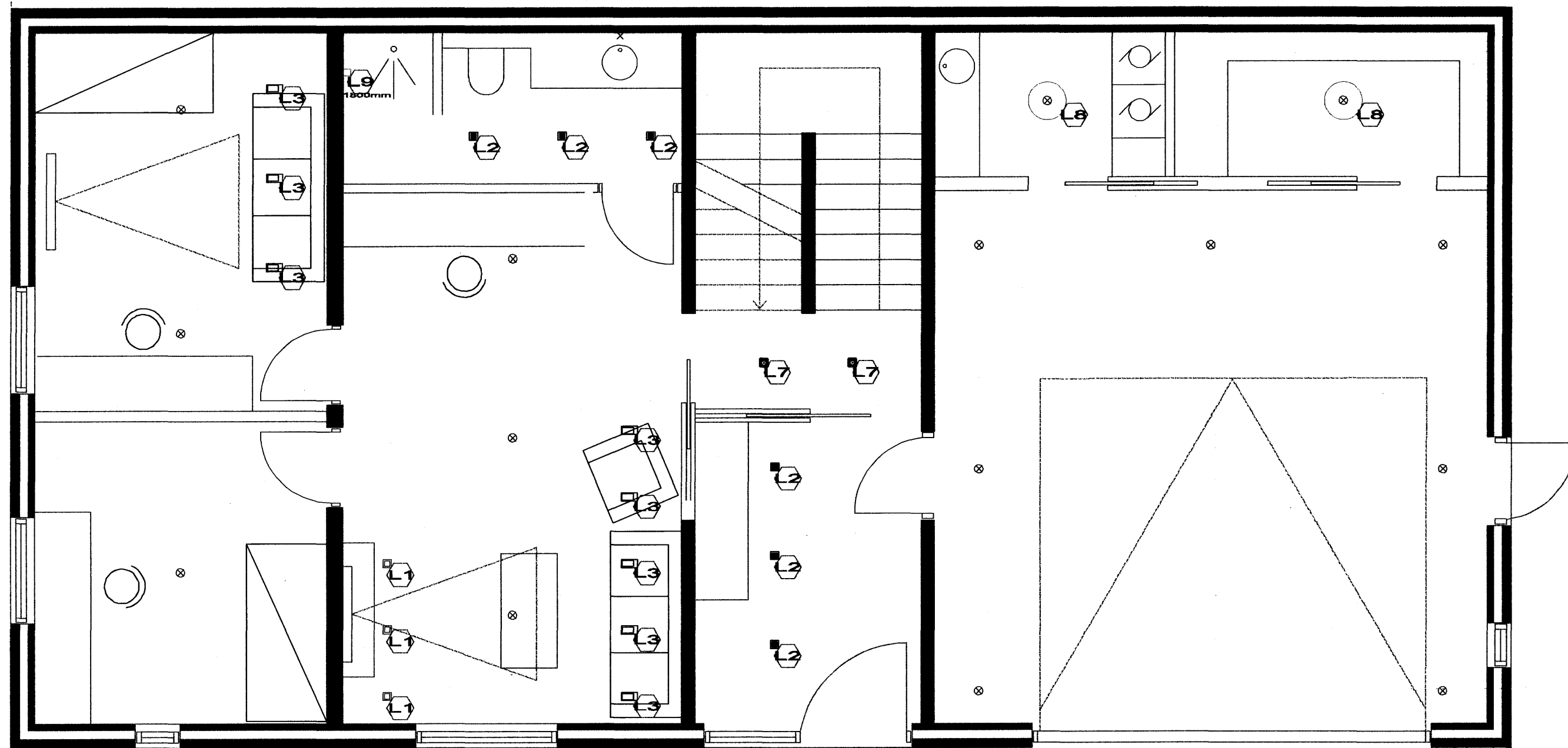
Grunnmynd - Lampaplan neðri hæð
