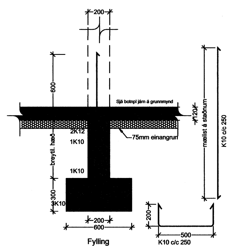
C Snið S01/B01 1:20
