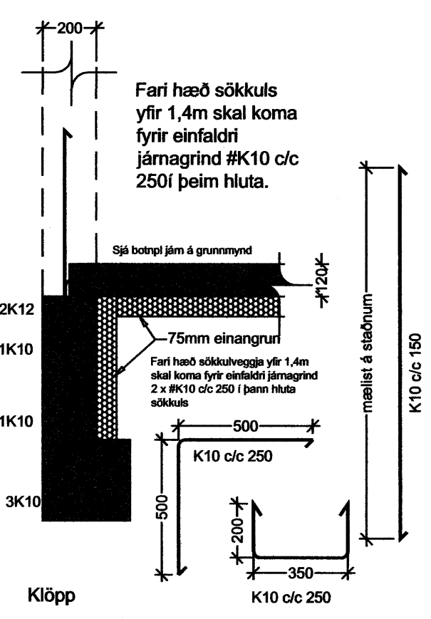
B Snið B01/B01 1:20
