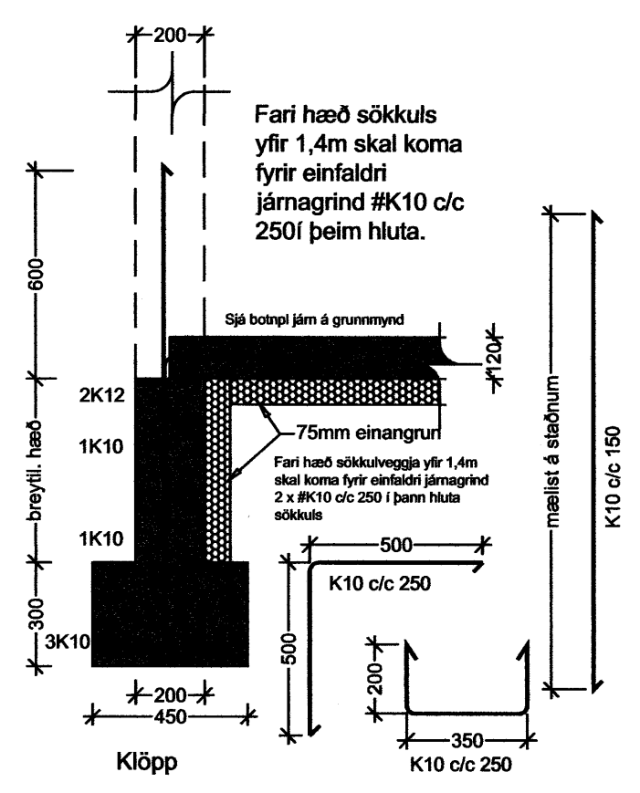
A Snið B01/B01 1:20
