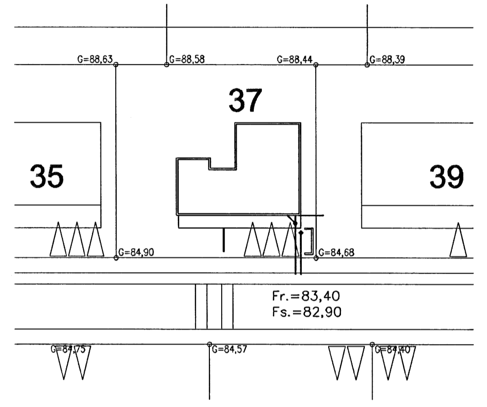
Afstöðumynd 1:500
