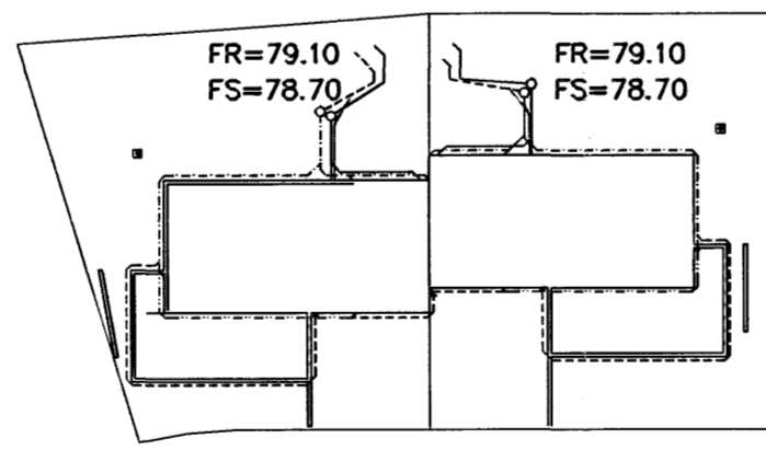
AFSTÖÐUMYND 1:50
