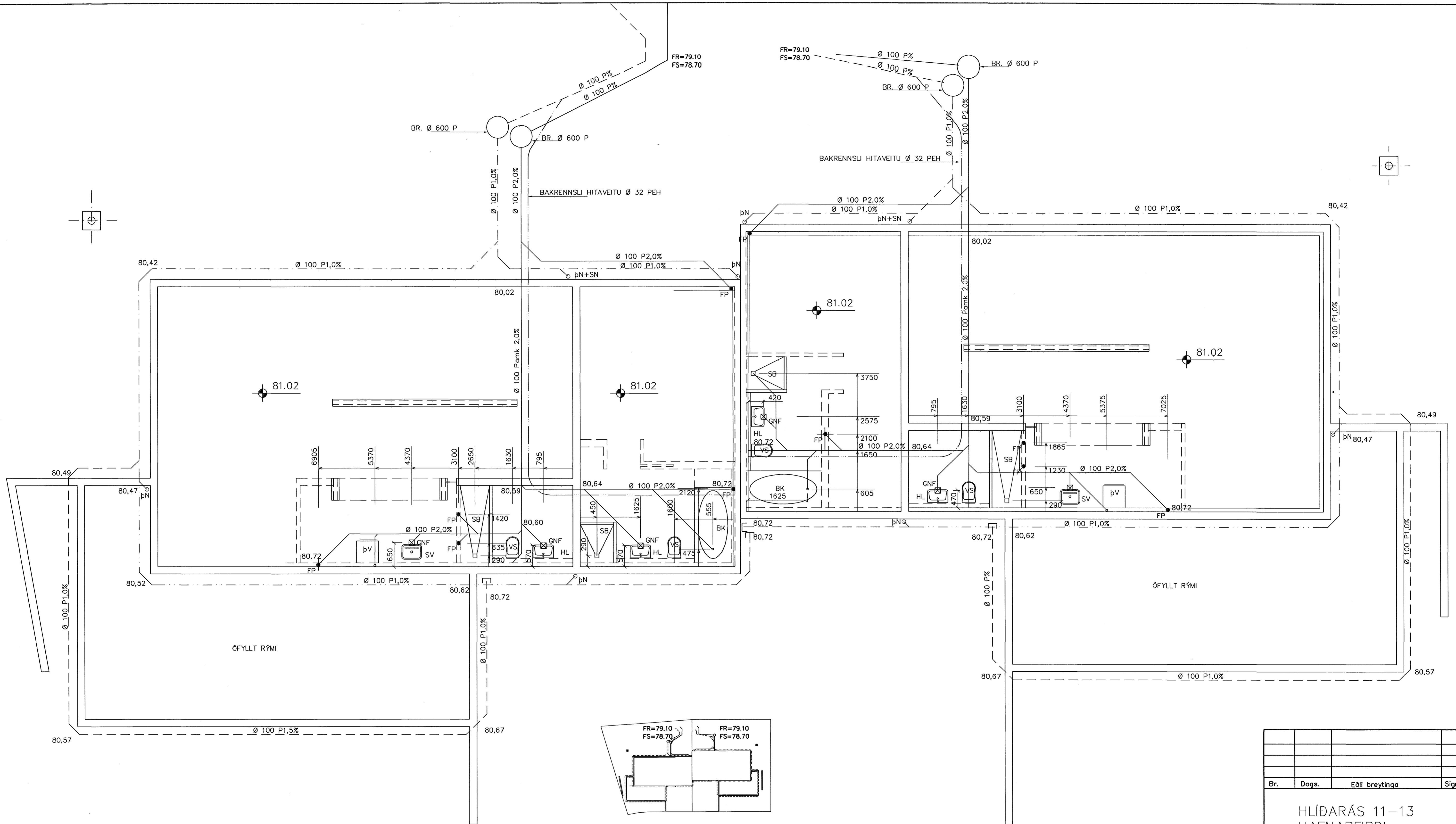
GRUNNMYND 1:50
