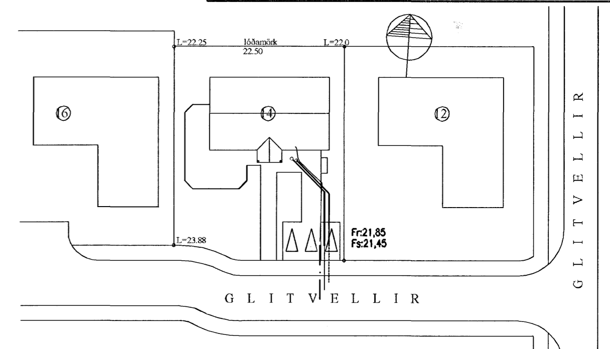
Afstöðumynd, 1:500
