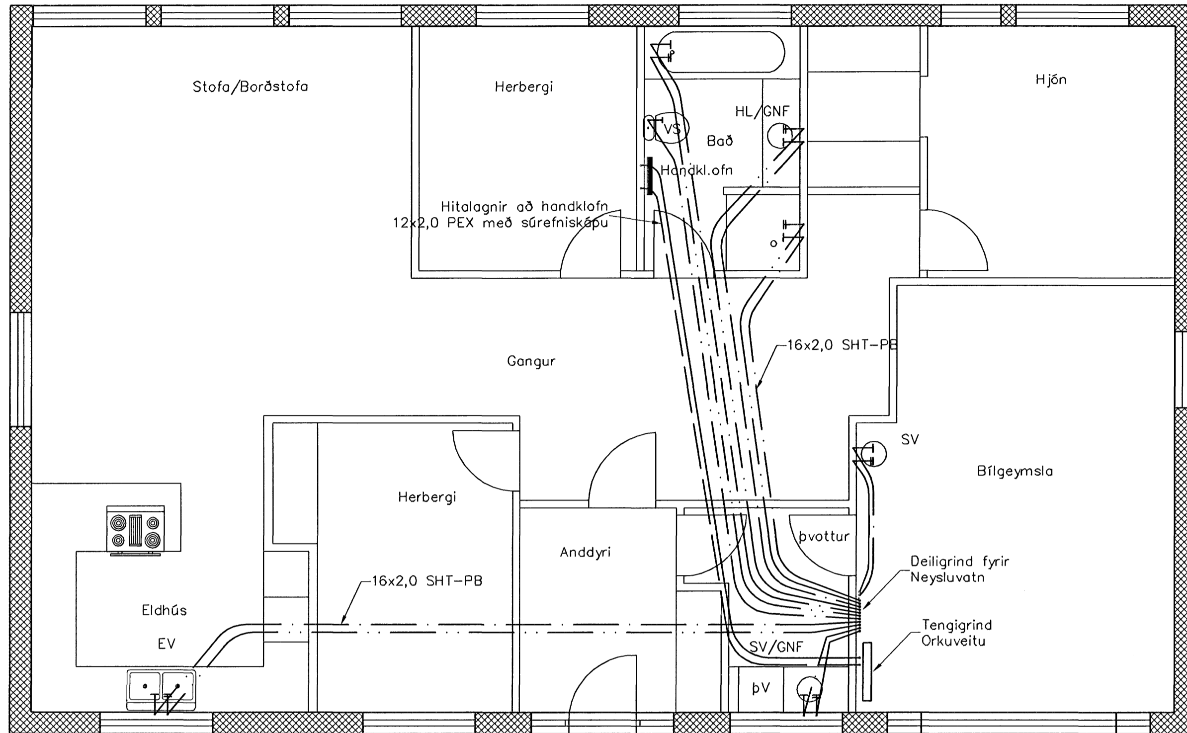
Neysluvatnslagnir. 1:50
