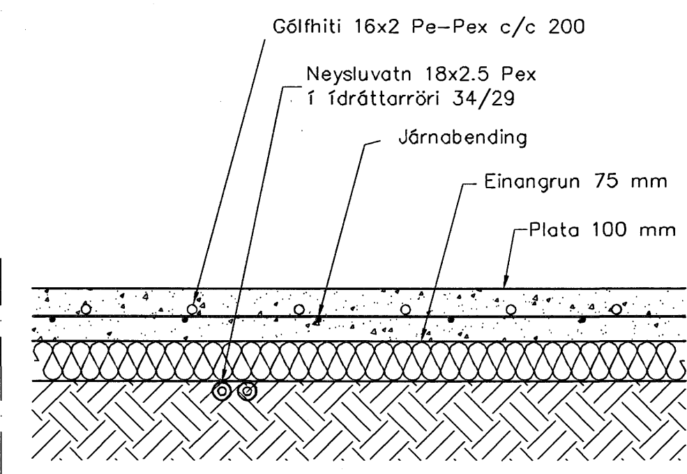
Hita- og vatnslagnir. Snið í botnplötu, bílgæmslu 1:10
