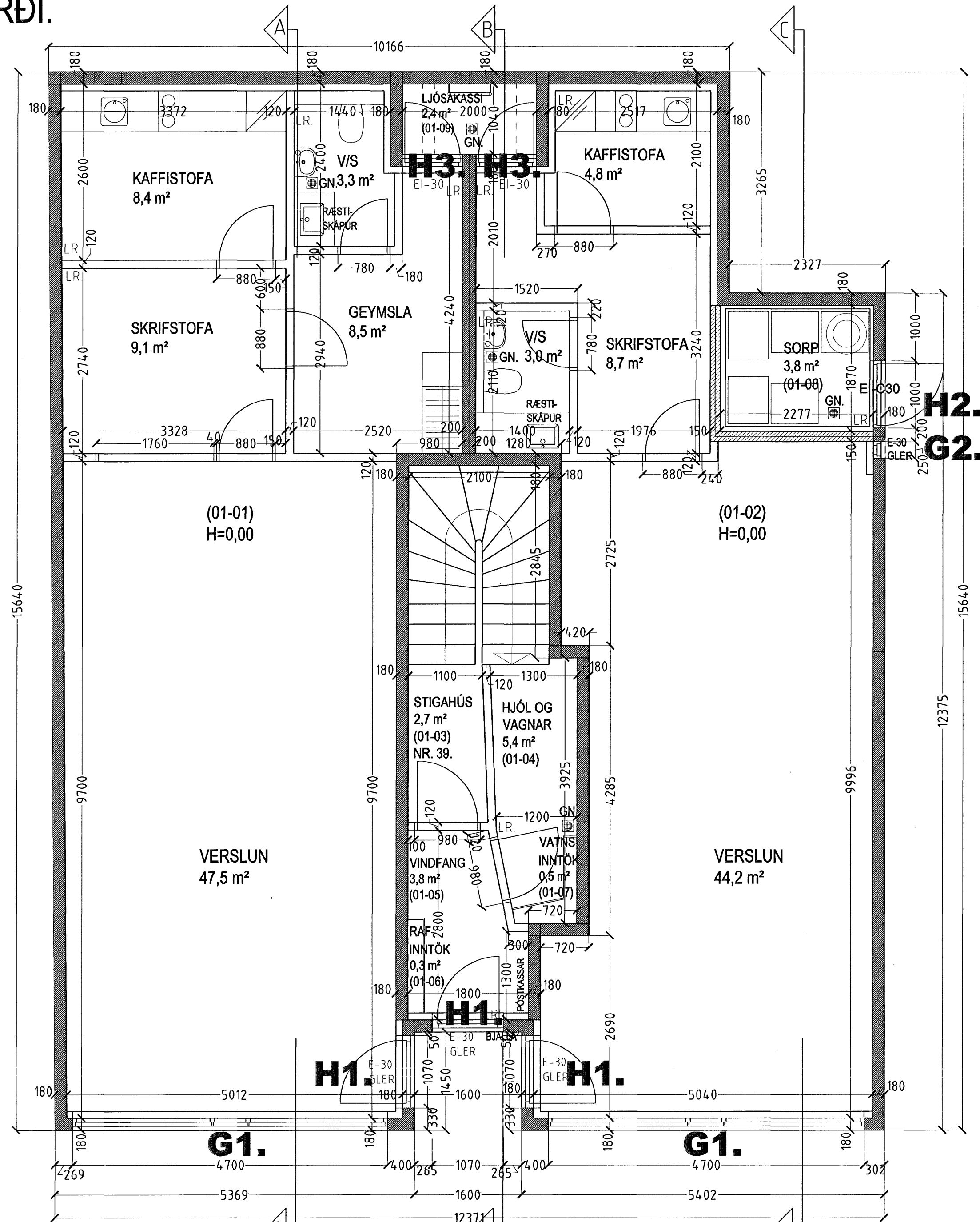
GRUNNMYND 1. HÆÐ MKV. 1:50.
