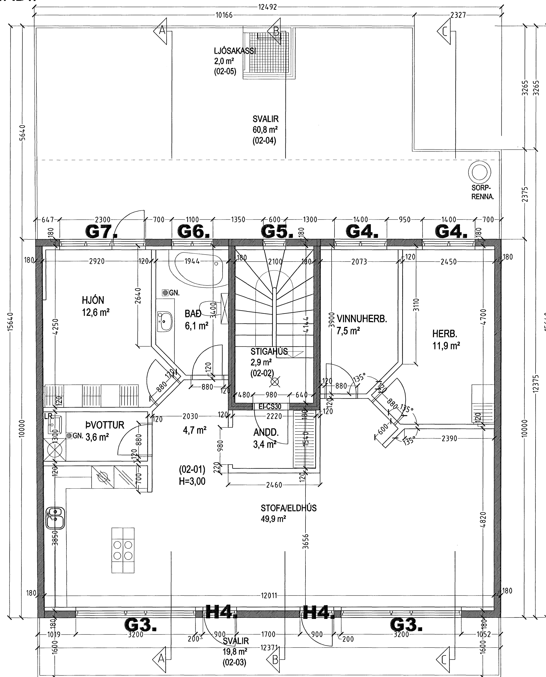
GRUNNMYND 2. HÆÐ MKV. 1:50.
