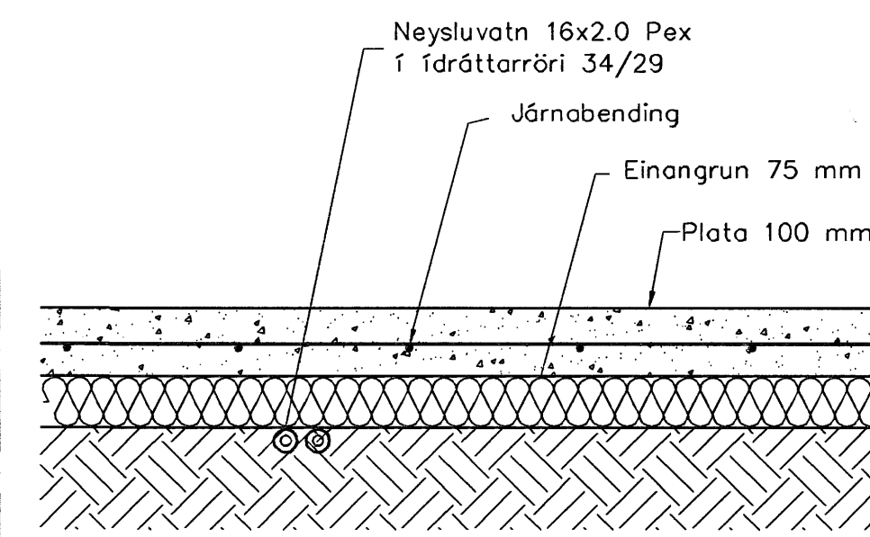
Hita- og vatnslagnir, Snið í botnplötu, bílgeymslu 1:10
