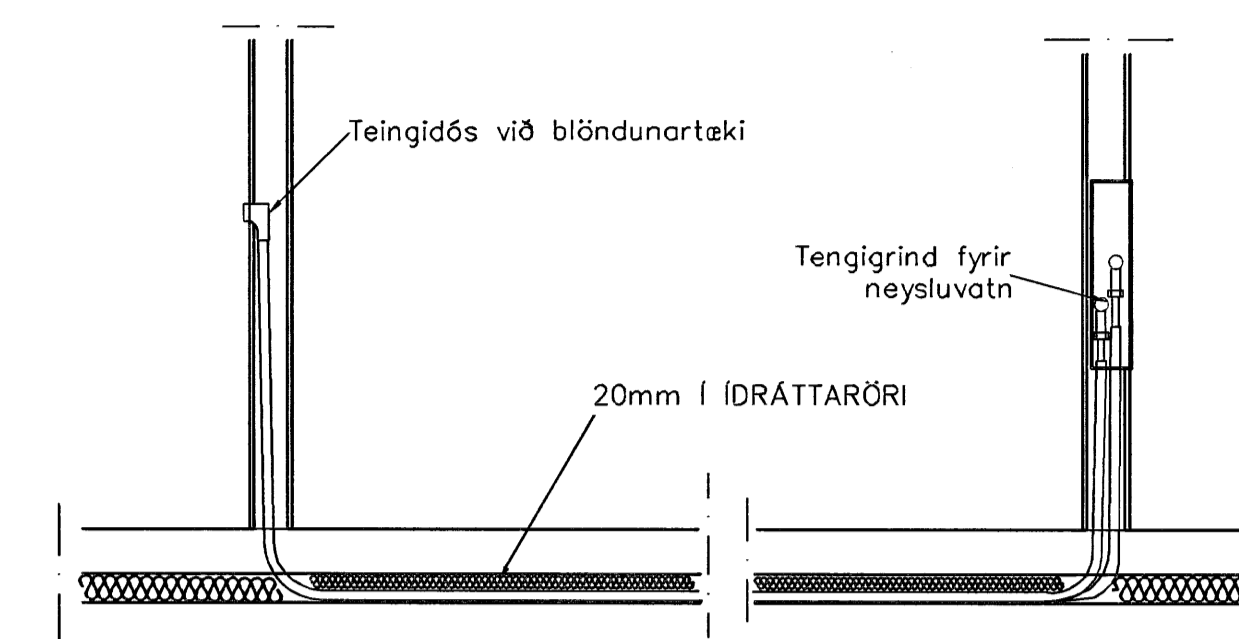
TENGING NEYSLUVATNSLAGNA 1:20
