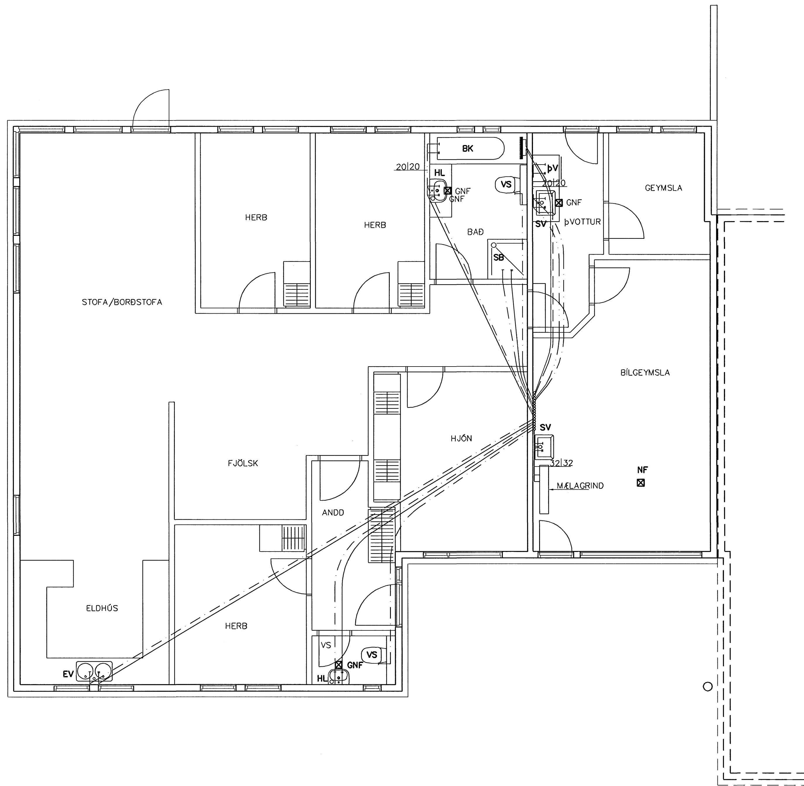
GRUNNMYND 1:50
