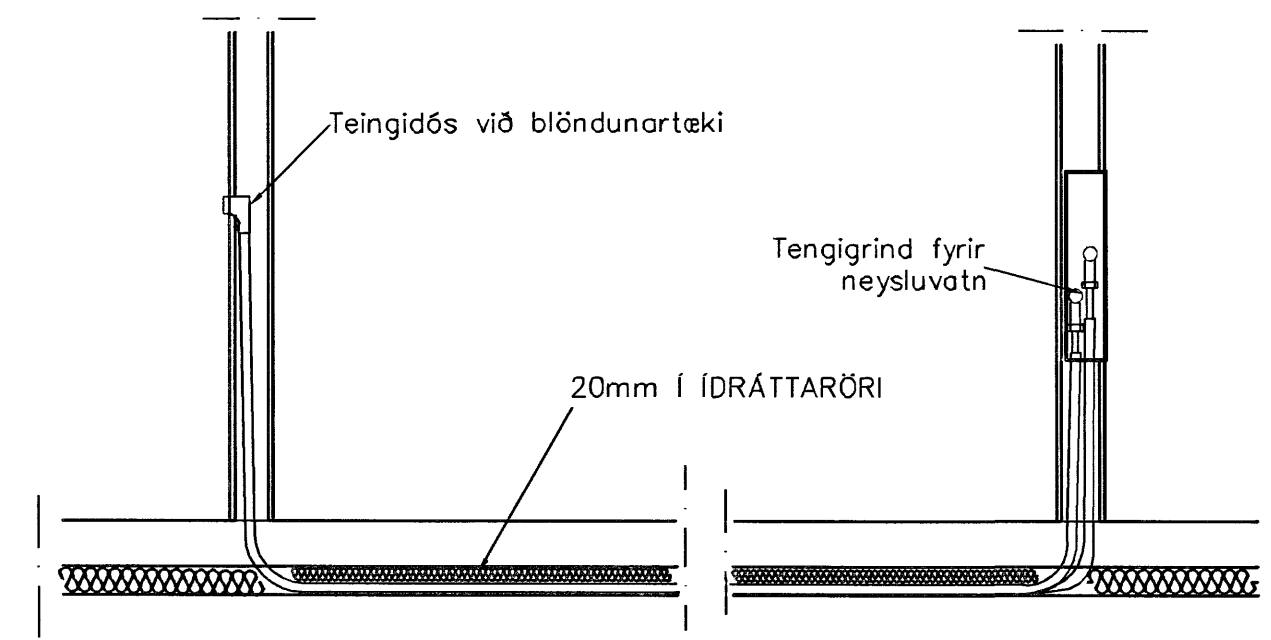
TENGING NEYSLUVATNSLAGNA 1:20
