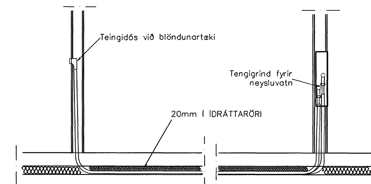
TENGING NEYSLUVATNSLAGNA 1:20
