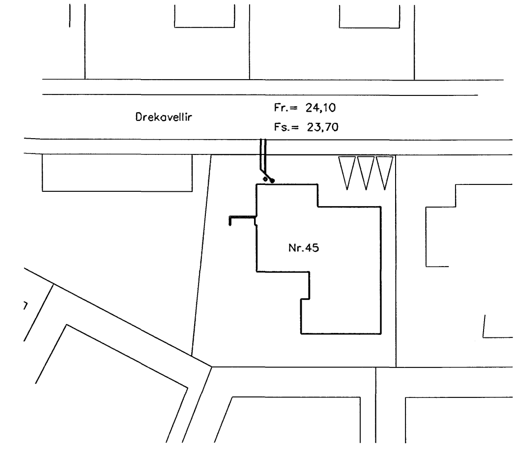
Afstöðmynd 1:500
