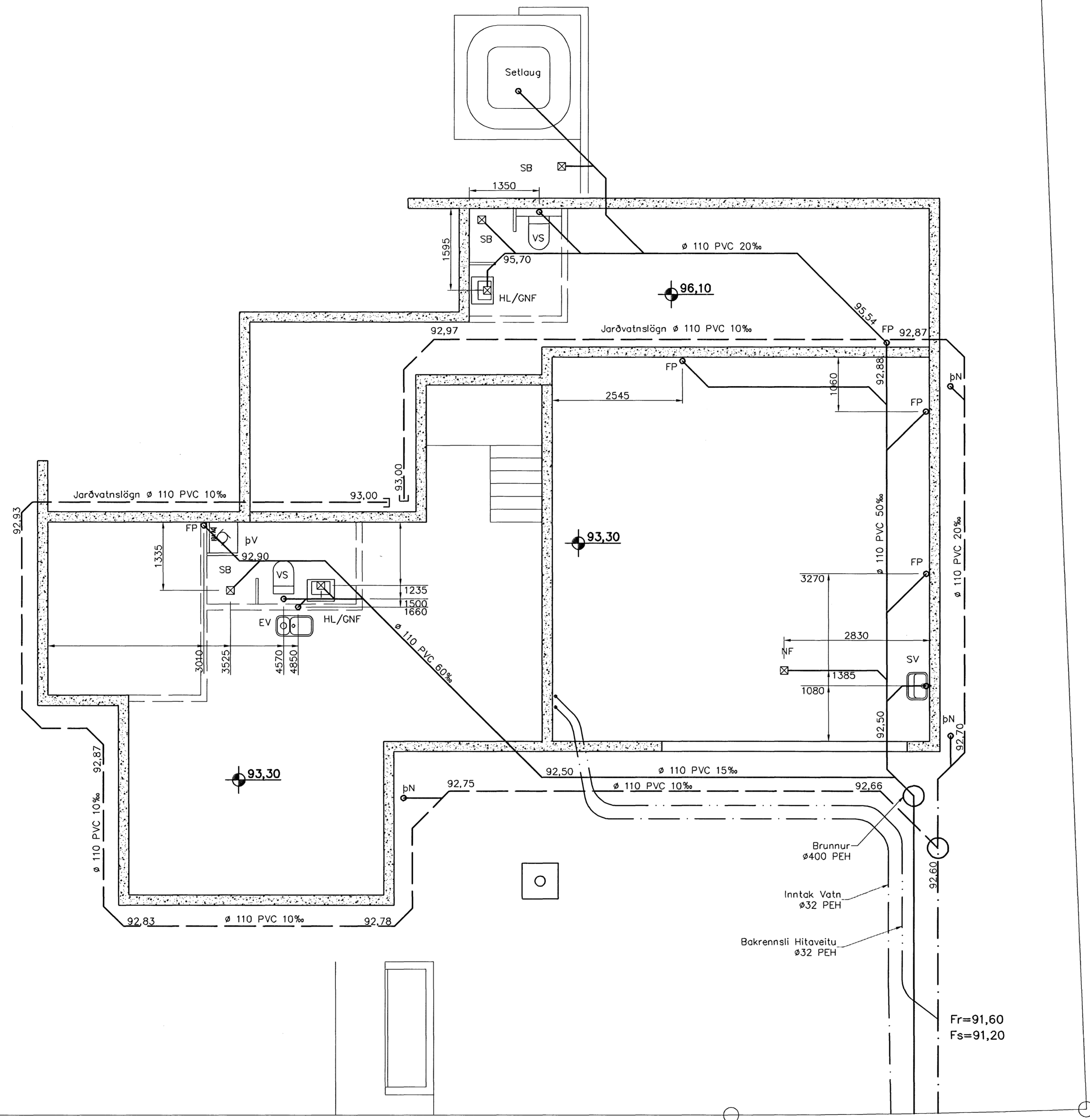
Grunnlagnir 1:50
