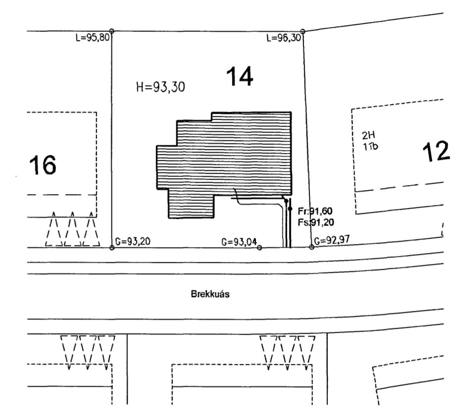
Afstöðumynd 1:500
