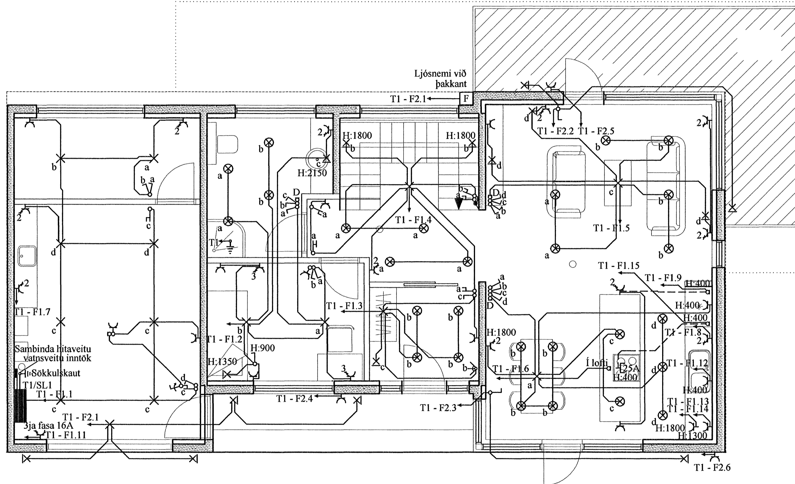
Grunnmynd - Raflögn efri hæðar
