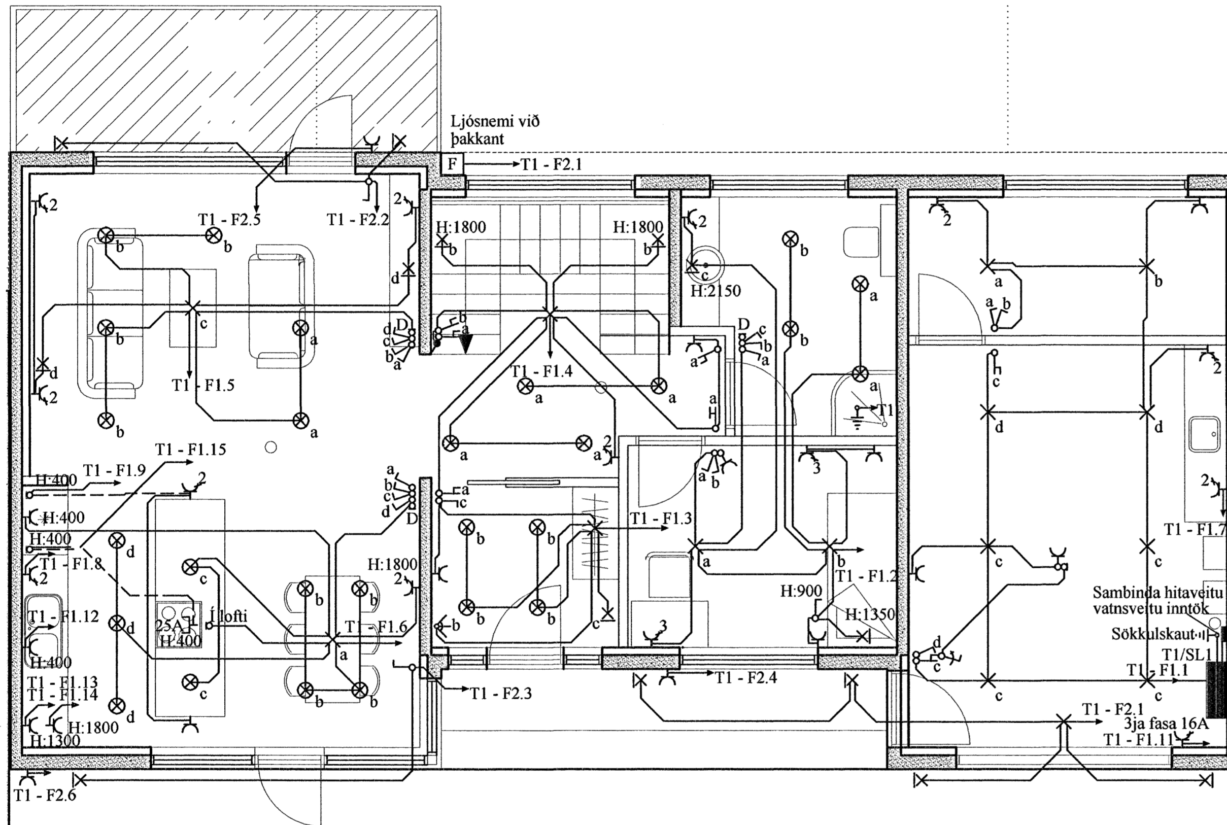
Grunnmynd - Raflögn efri hæðar
