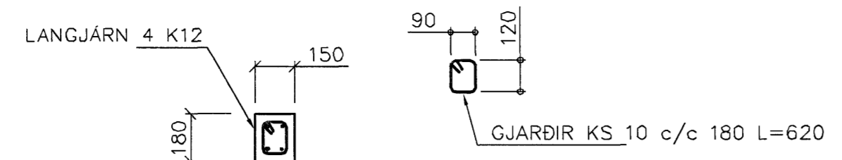
SÚLA S3 1:20
