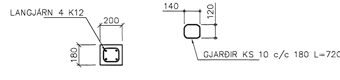
SÚLA S2 1:20
