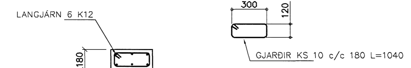
SÚLA S4 1:20
