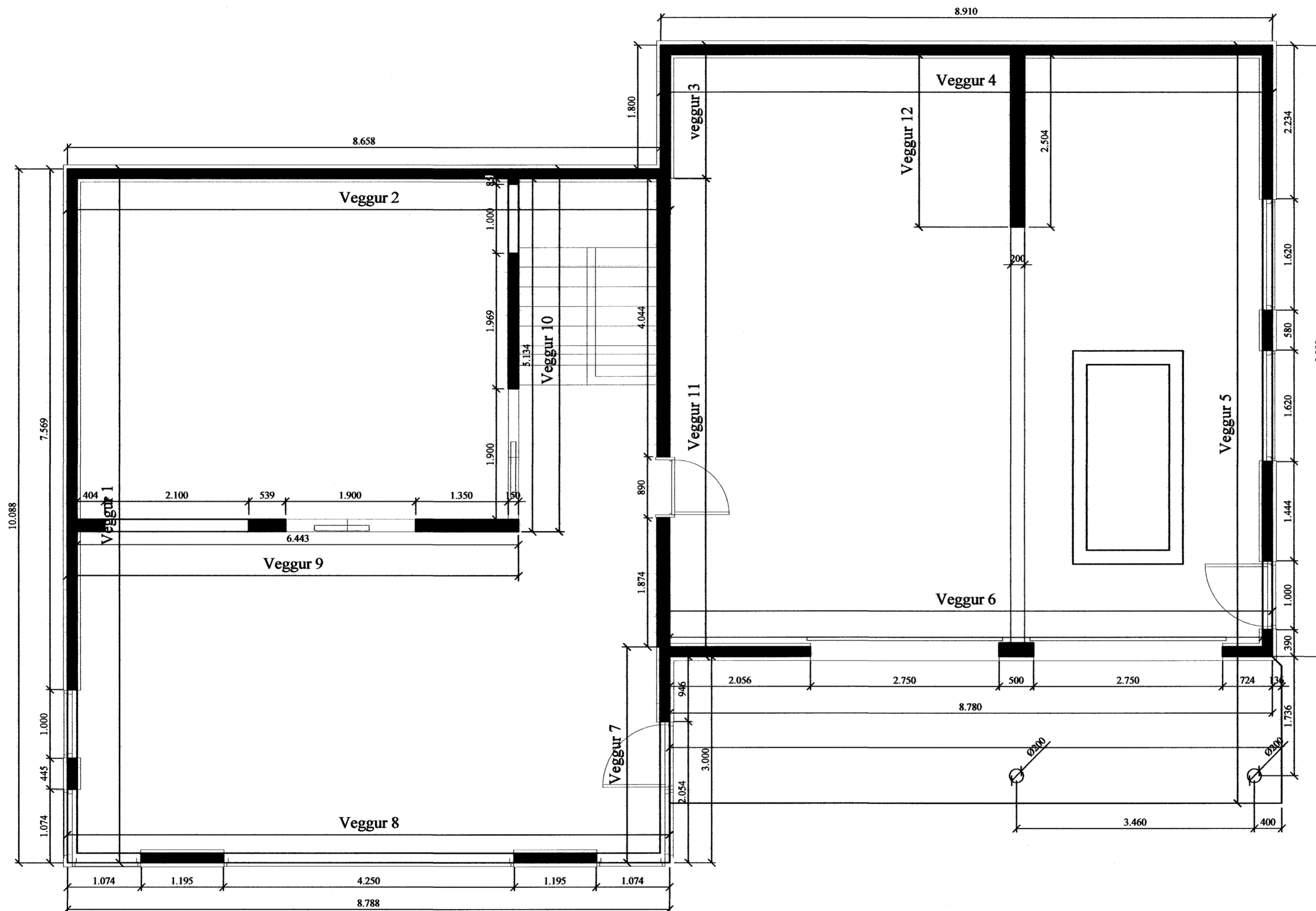
Grunnmynd 1. hæðar
