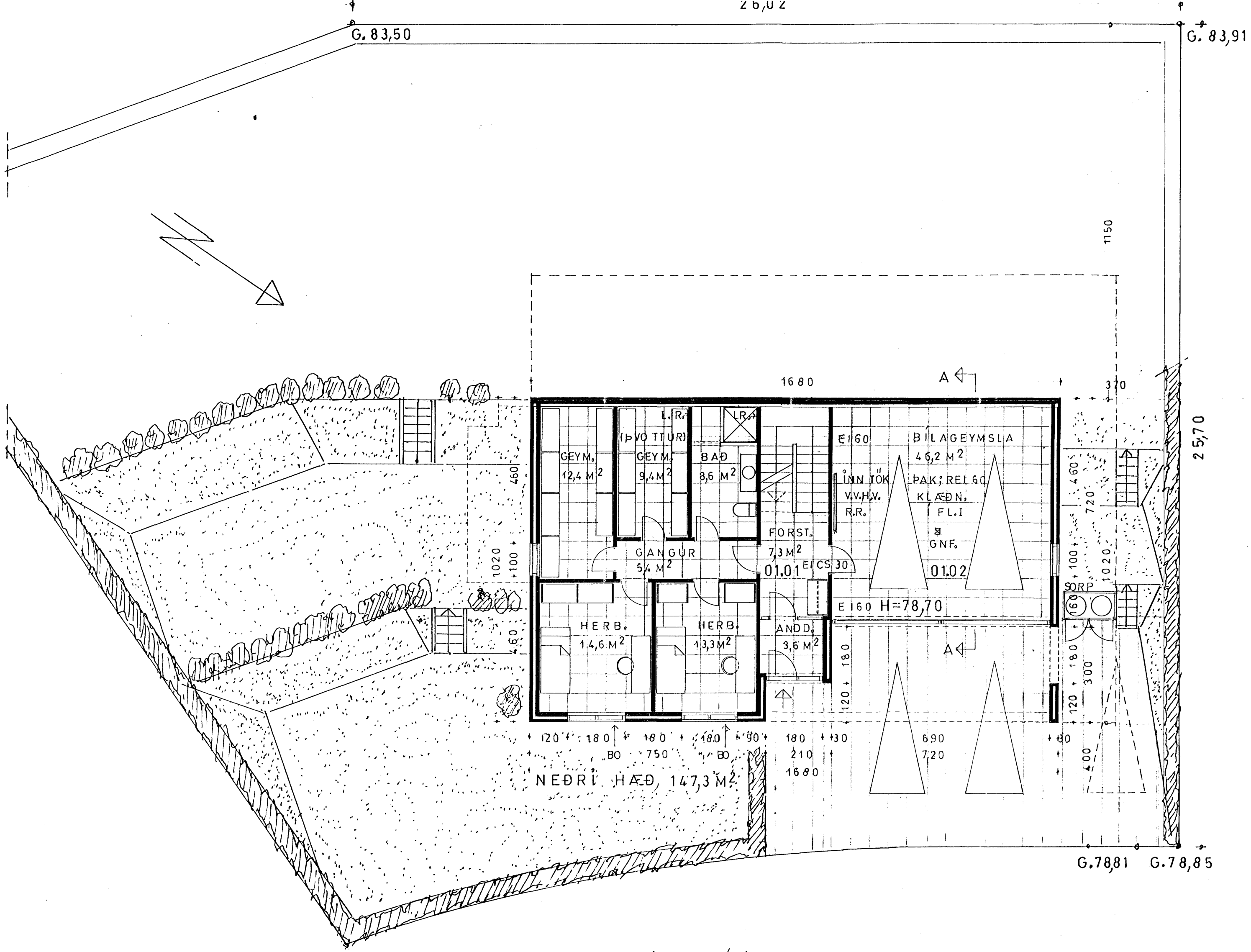
AFSTÖÐUMYND, M.1:500
