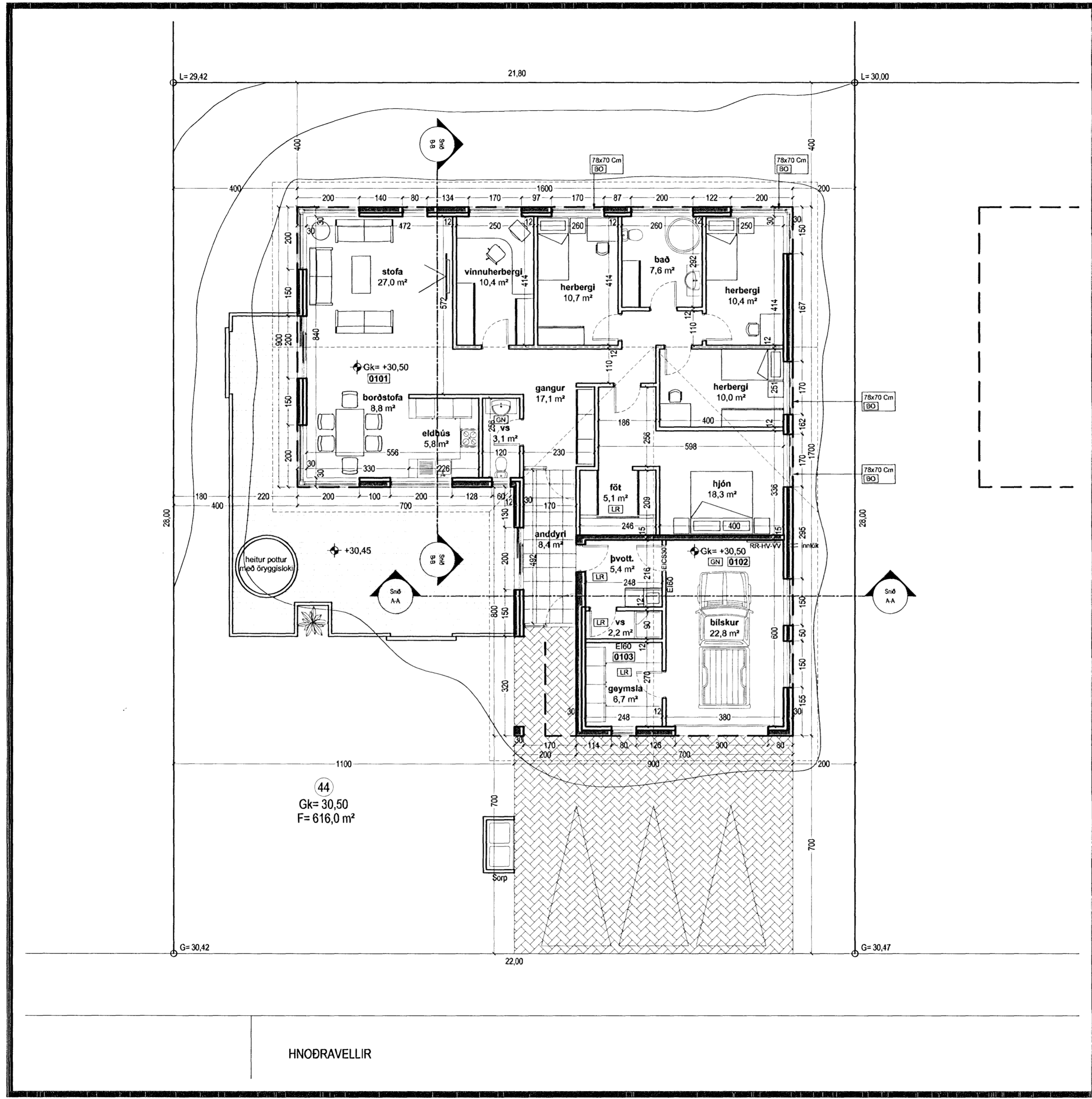
Grunnmynd 1:100
