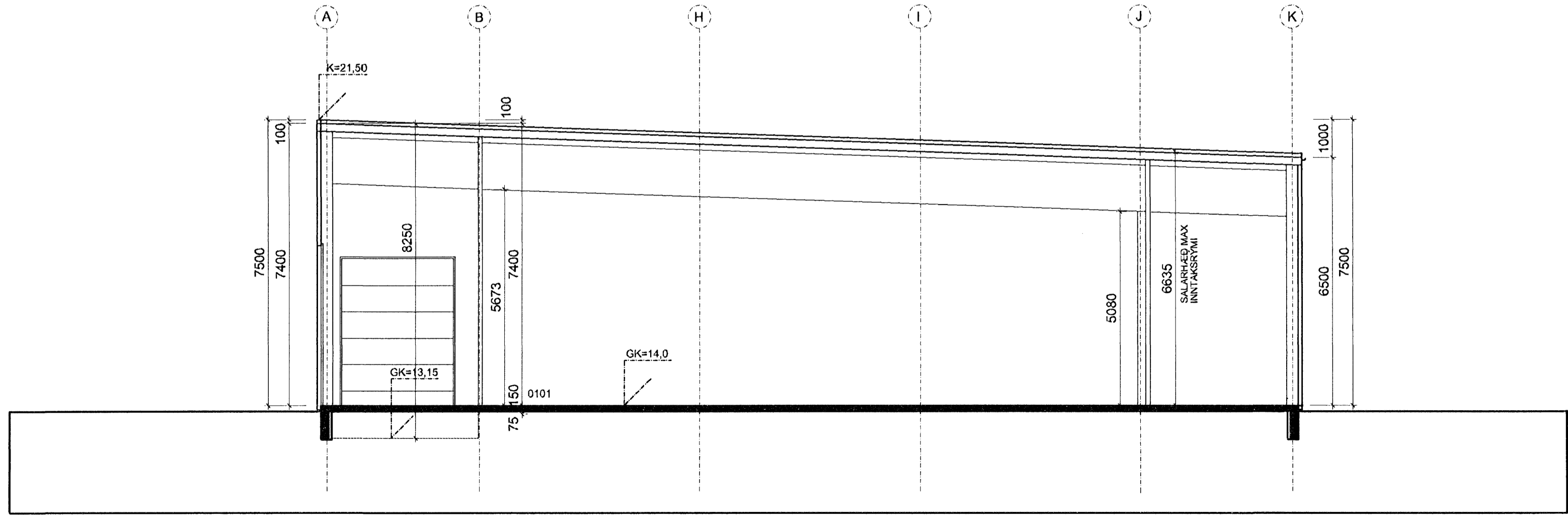
SNEIÐING B-B, M: 1/100,
