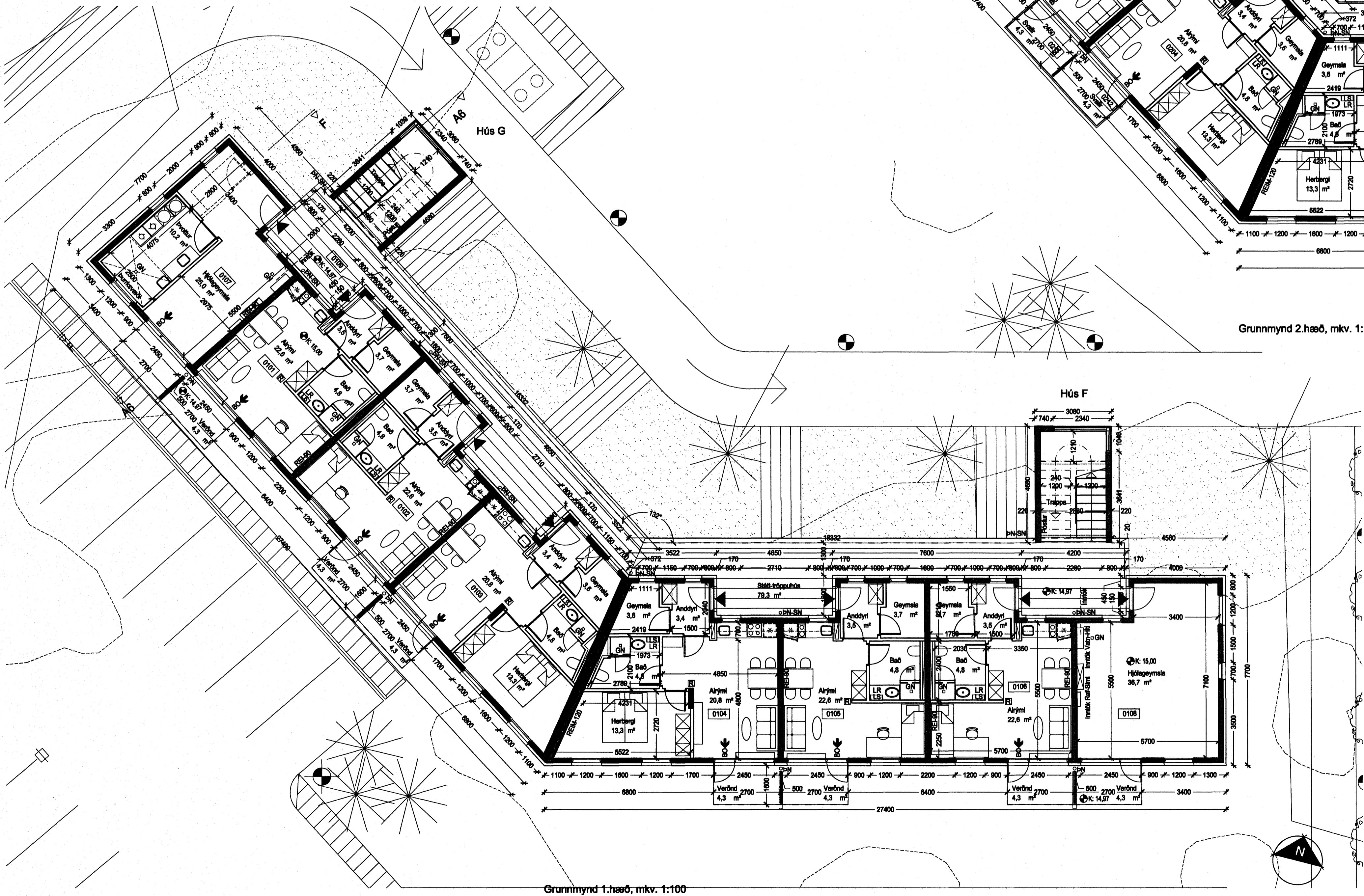
Grunnmynd 1.hæð, mkv. 1:100 L60 skv. uppdrætti landslagsarkitekt
