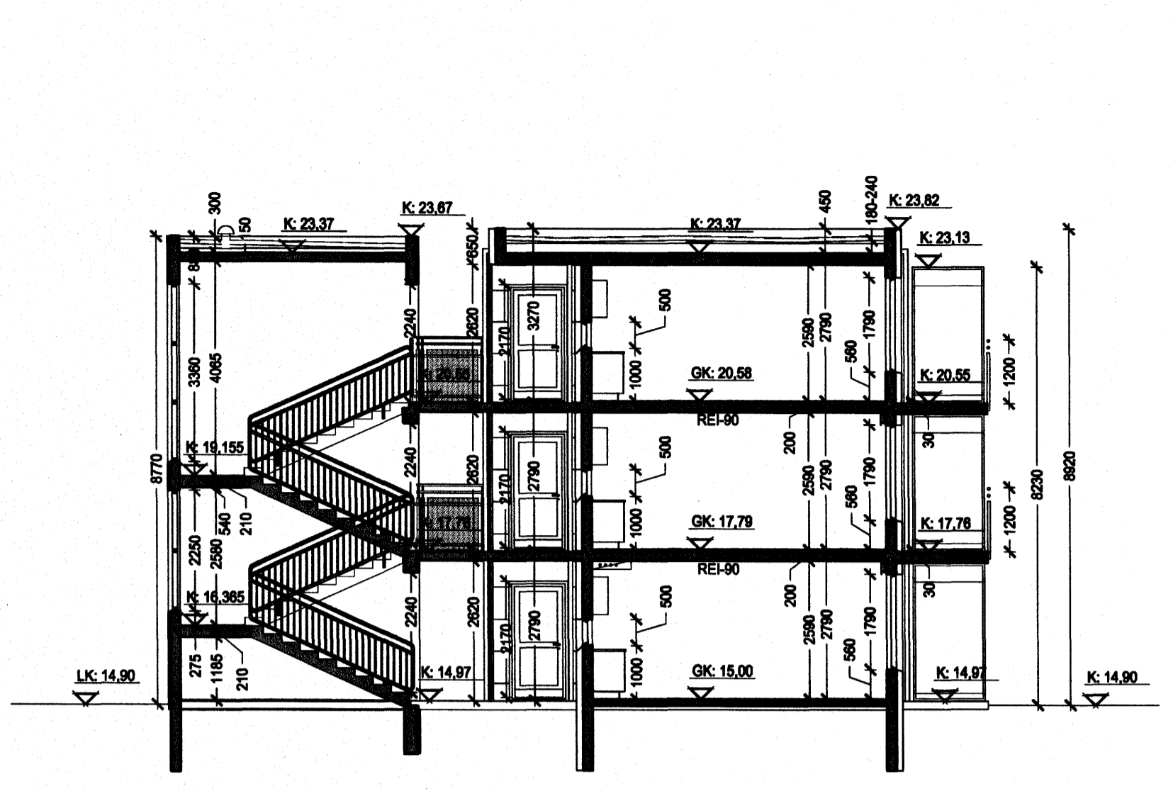
Sneiðing A6-A6, mkv. 1:100
