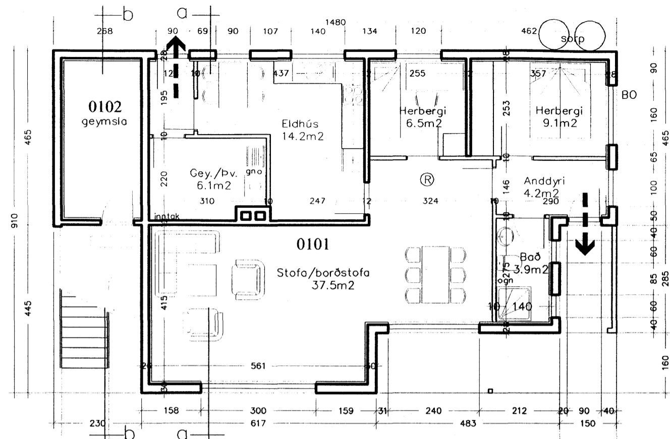
Grunnmynd 1.hæð 1:100
