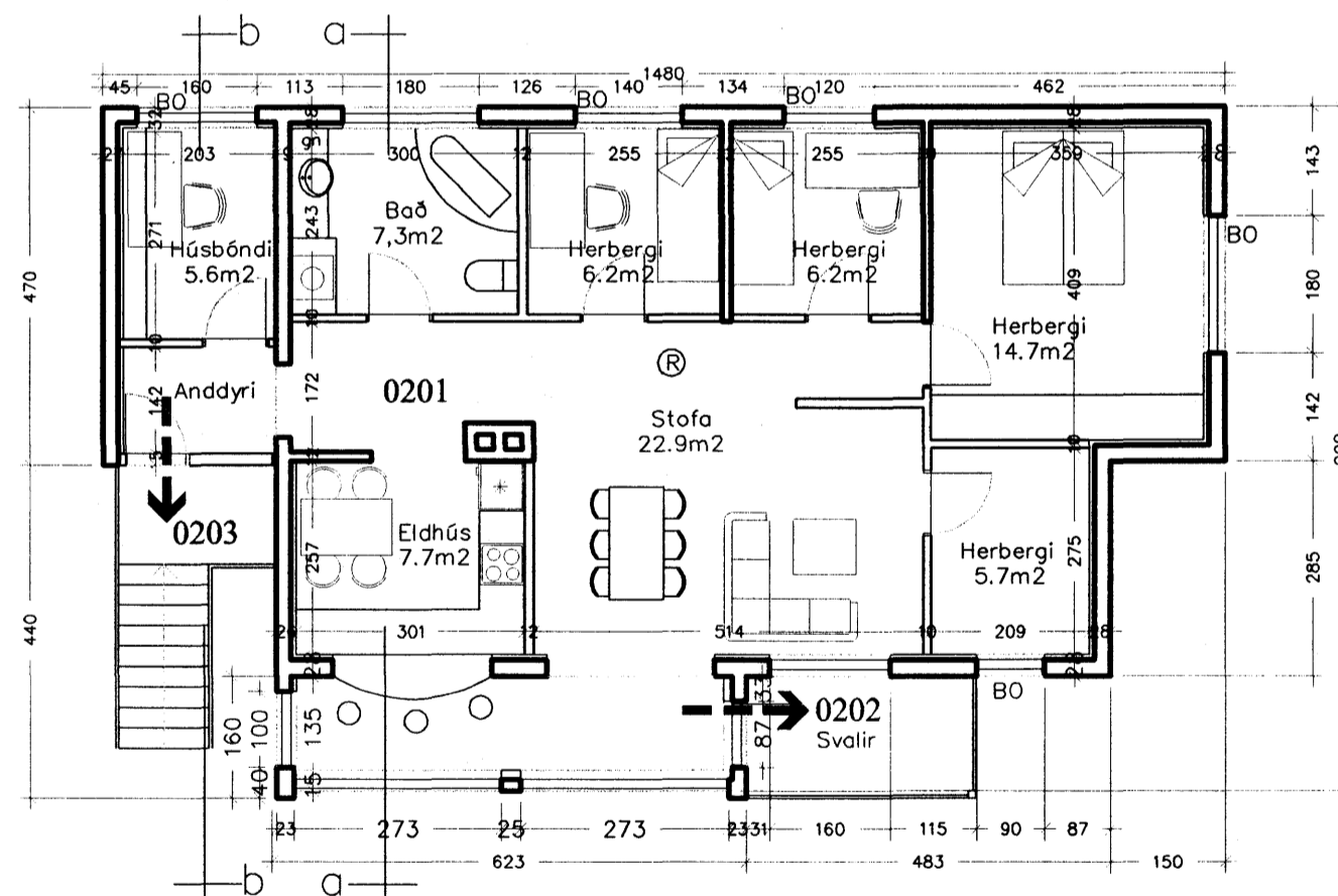
Grunnmynd 2.hæð 1:100
