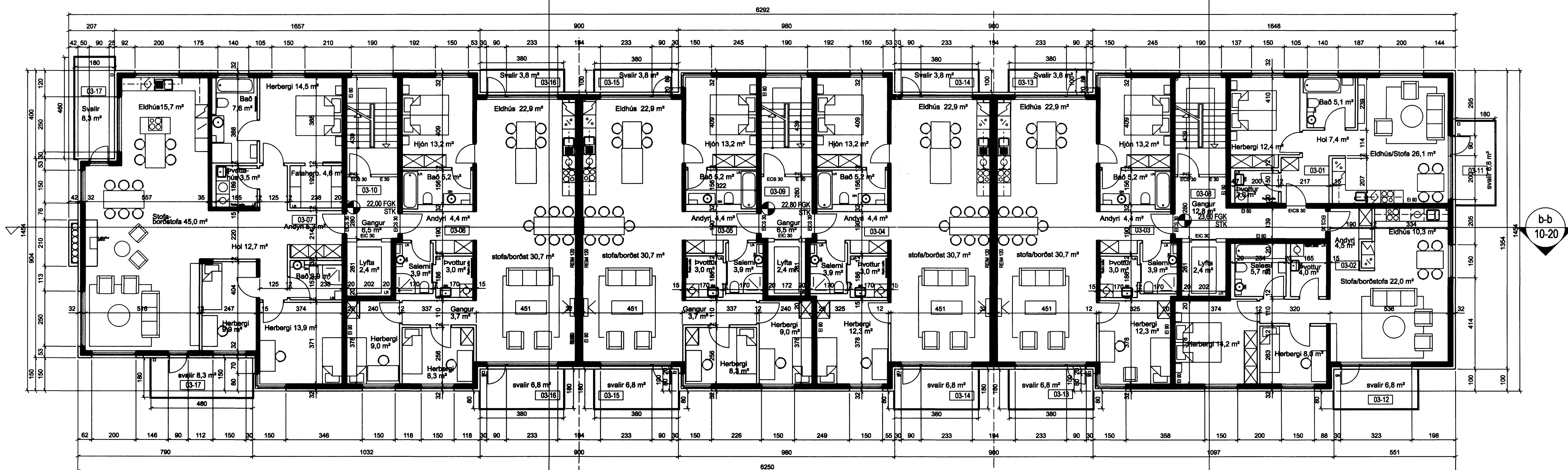
GRUNNMYND 3. HÆÐ 1:100
