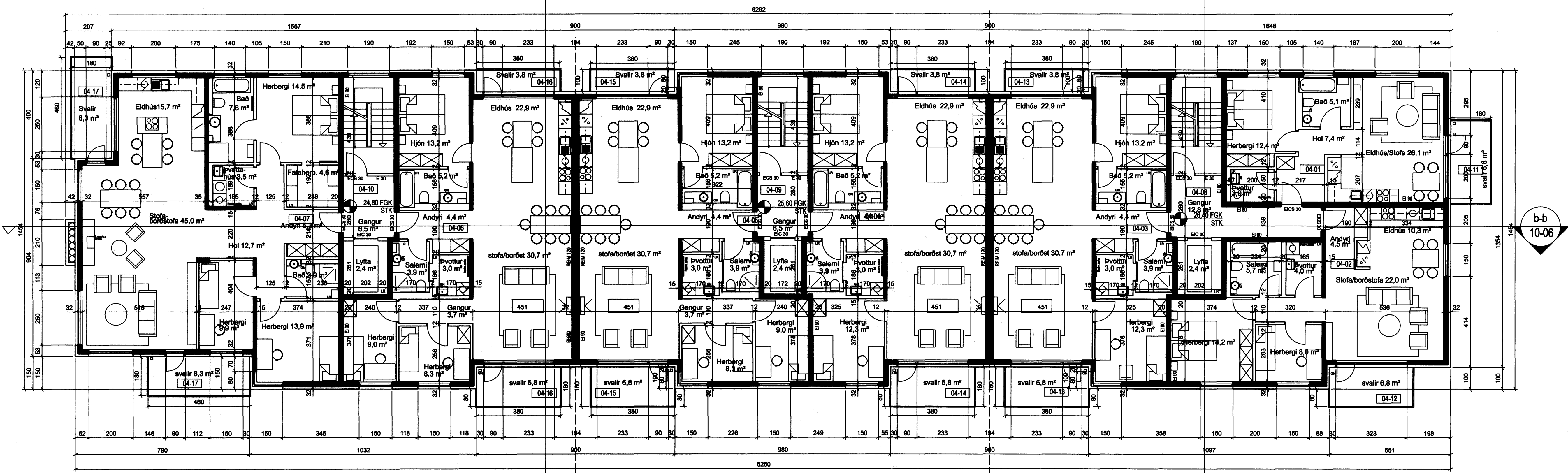
GRUNNMYND 4. HÆÐ 1:100
