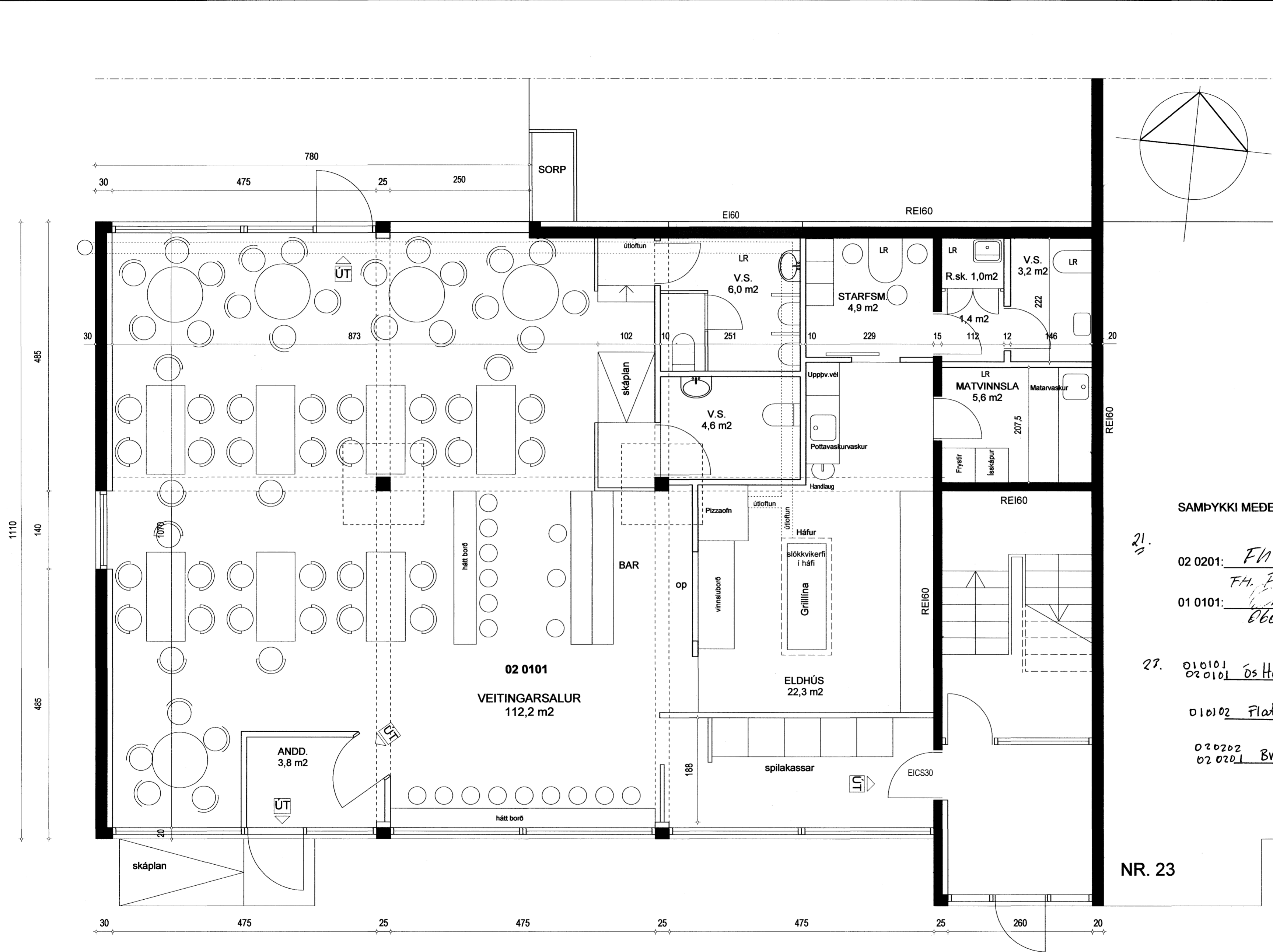
GRUNNMYD JARÐHÆÐAR 1.50
