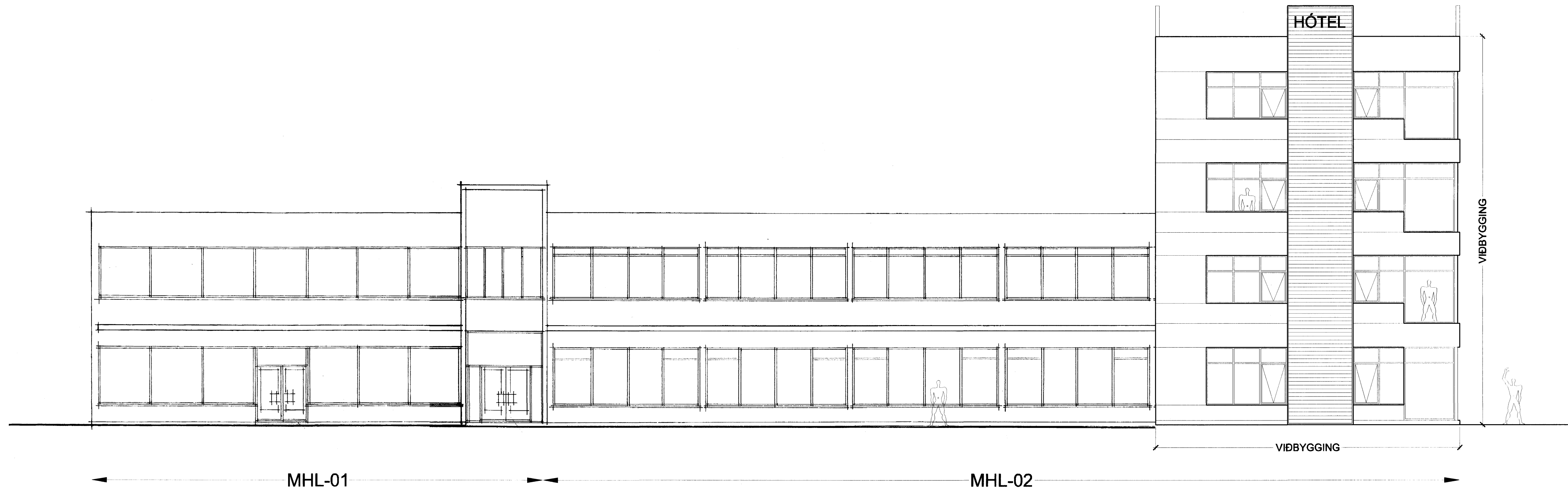
SUÐURÚTLIT
