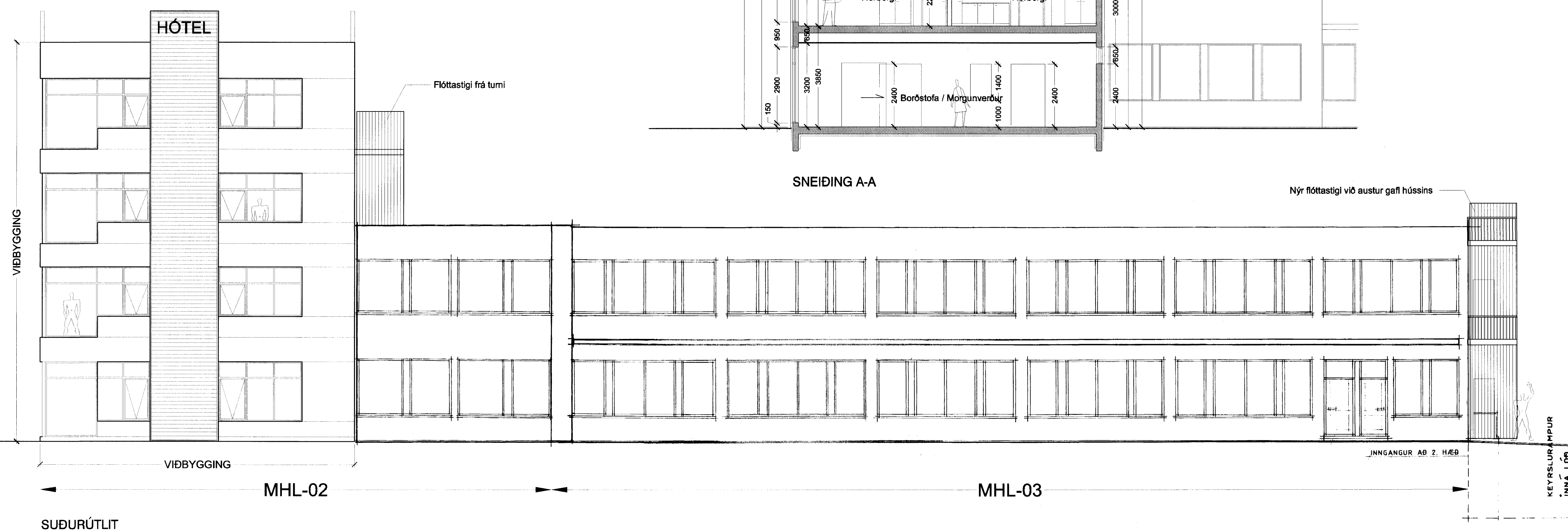
SUÐURÚTLIT
