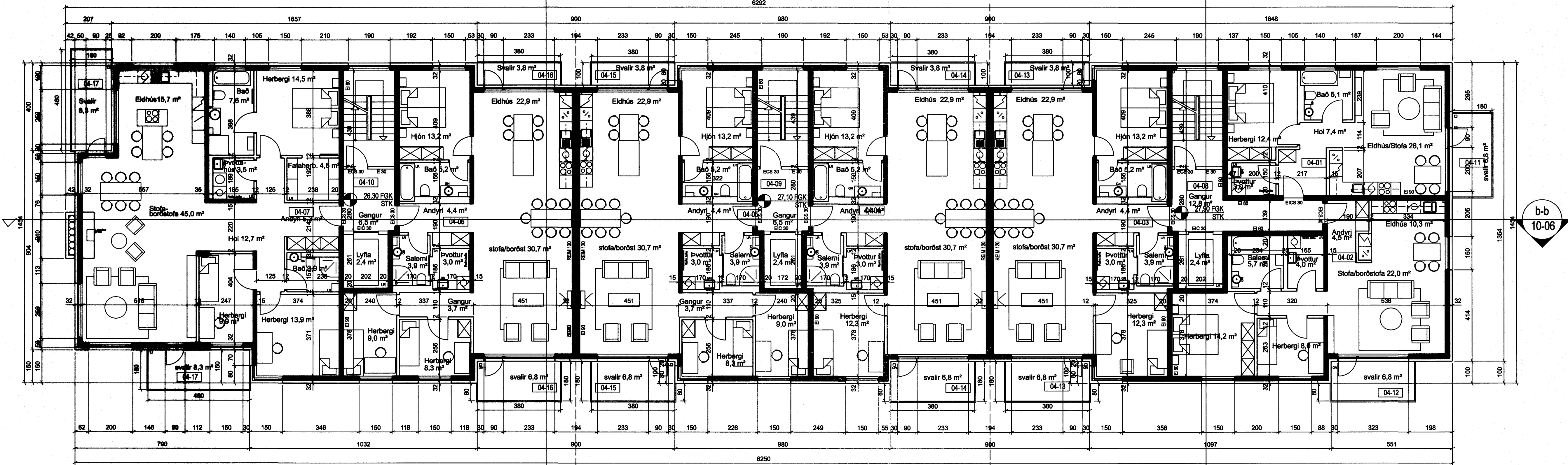
GRUNNMYND 4. HÆÐ 1:100
