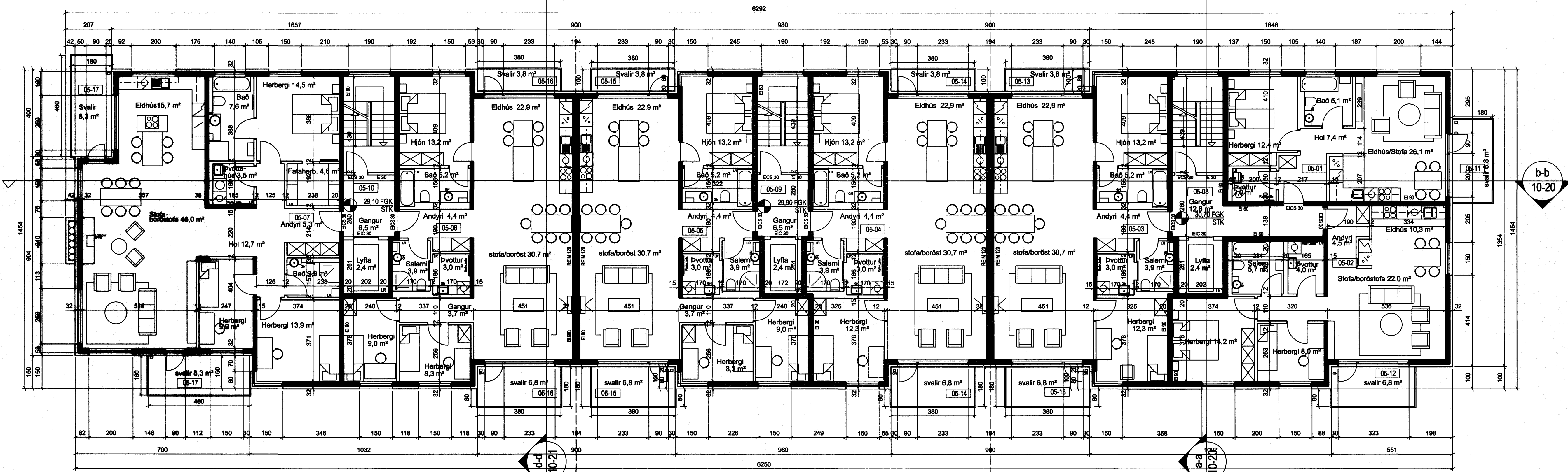
GRUNNMYND 5. HÆÐ 1:100
