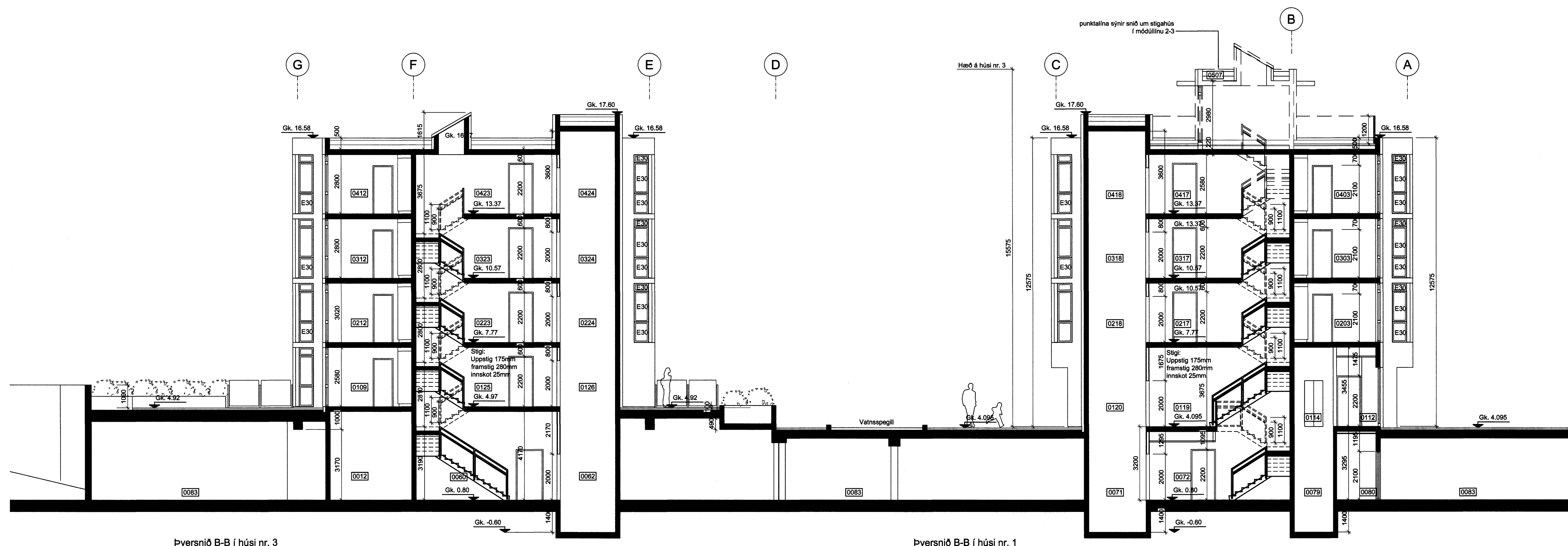
Þversnið B-B í húsi nr. 3
