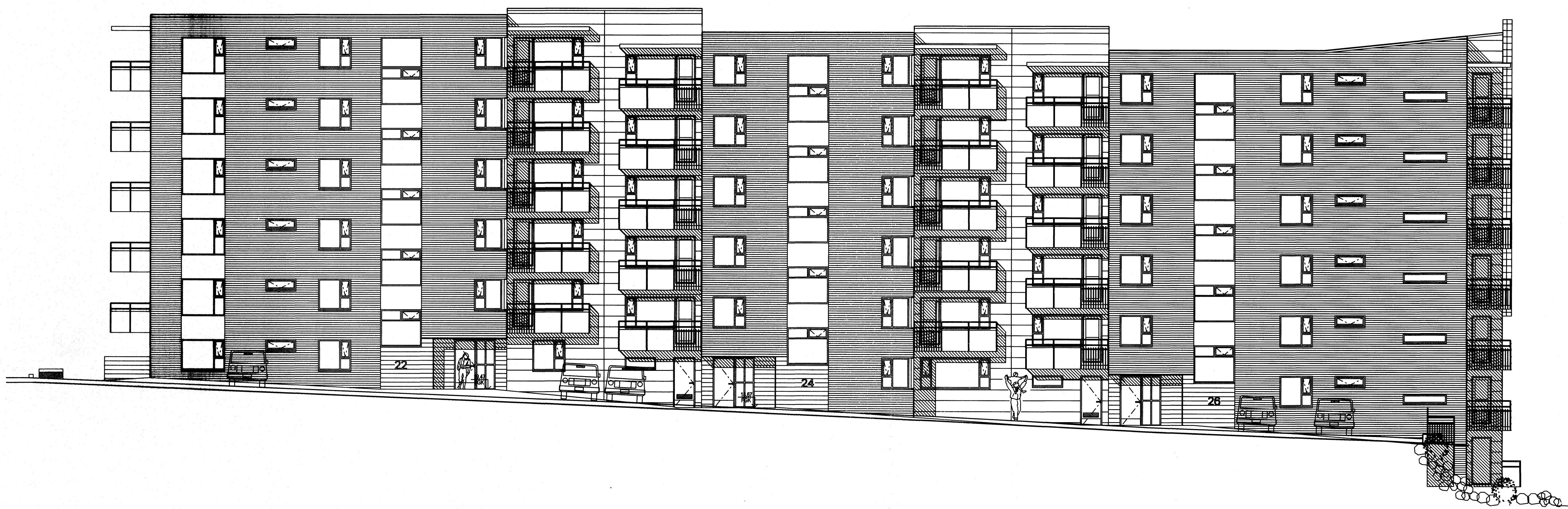
ÚTLIT 1:100 Norð-austur hlið
