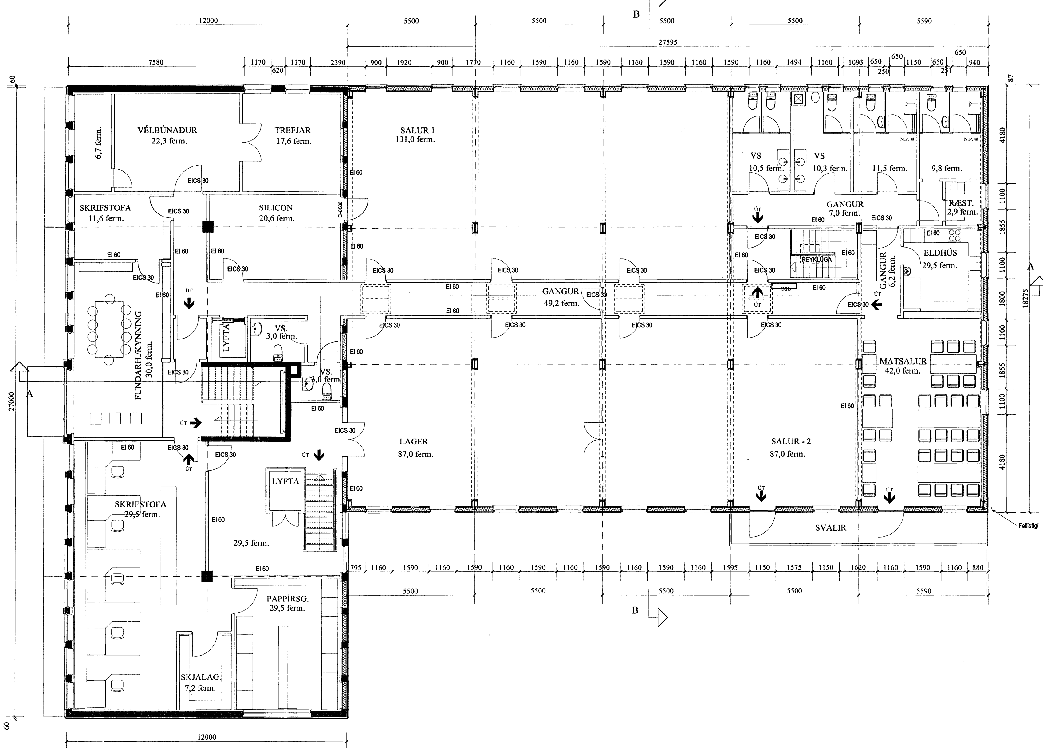
GRUNNMYND 2. HÆÐ
