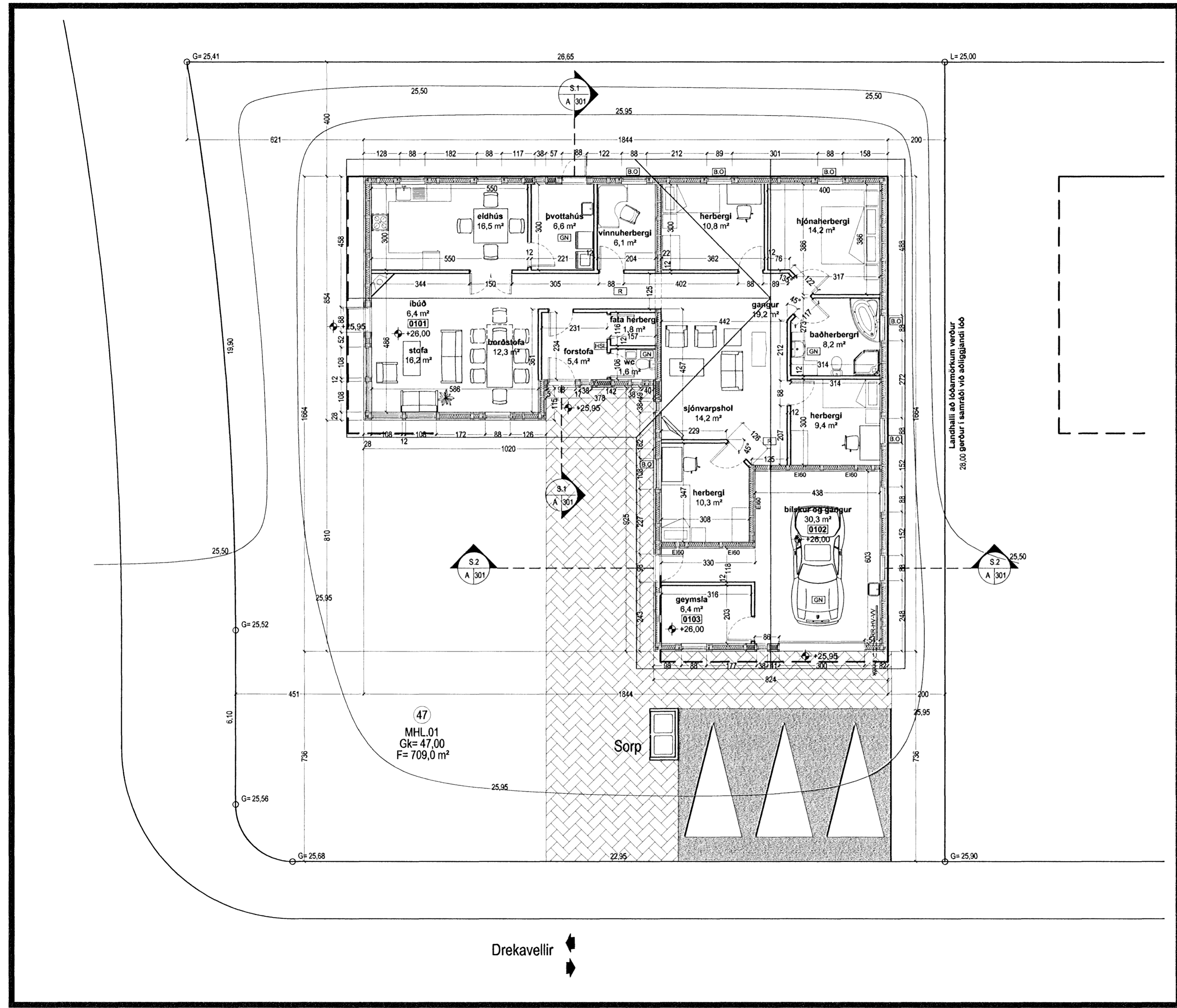
Grunnmynd 1:100
