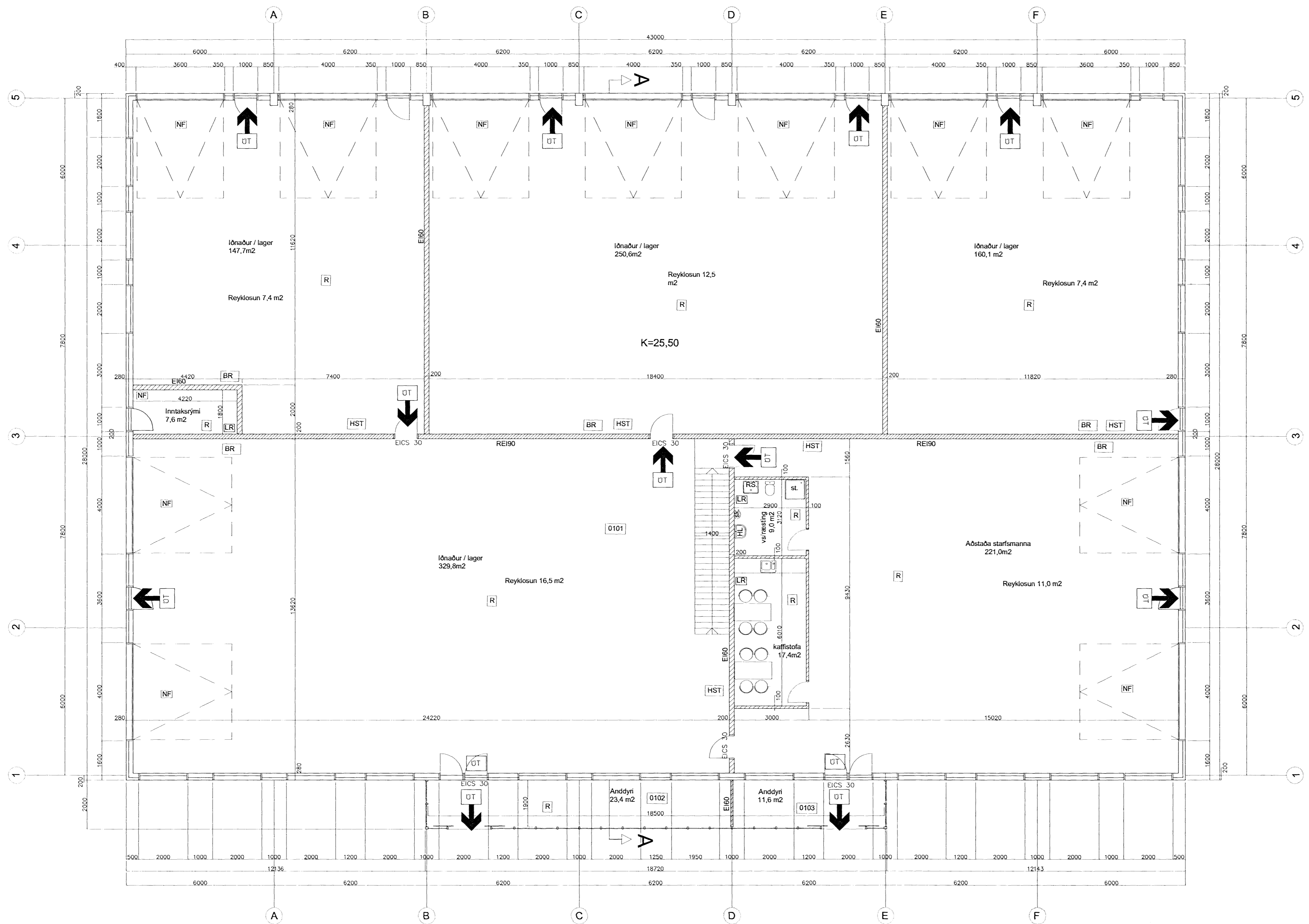
Grunnmynd 1. hæðar 1:100
