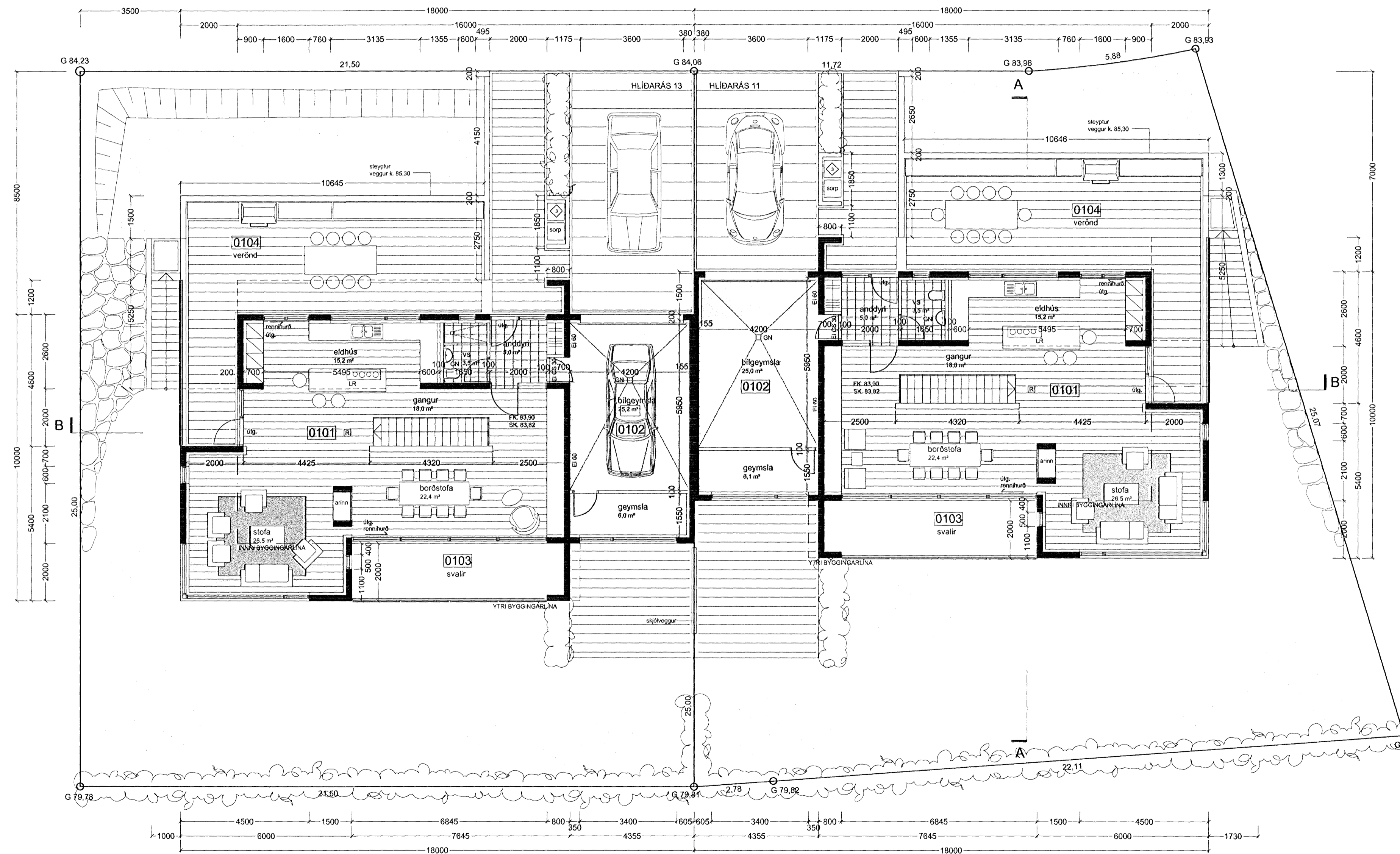
GRUNNMYND EFRI HÆÐ M 1:100
