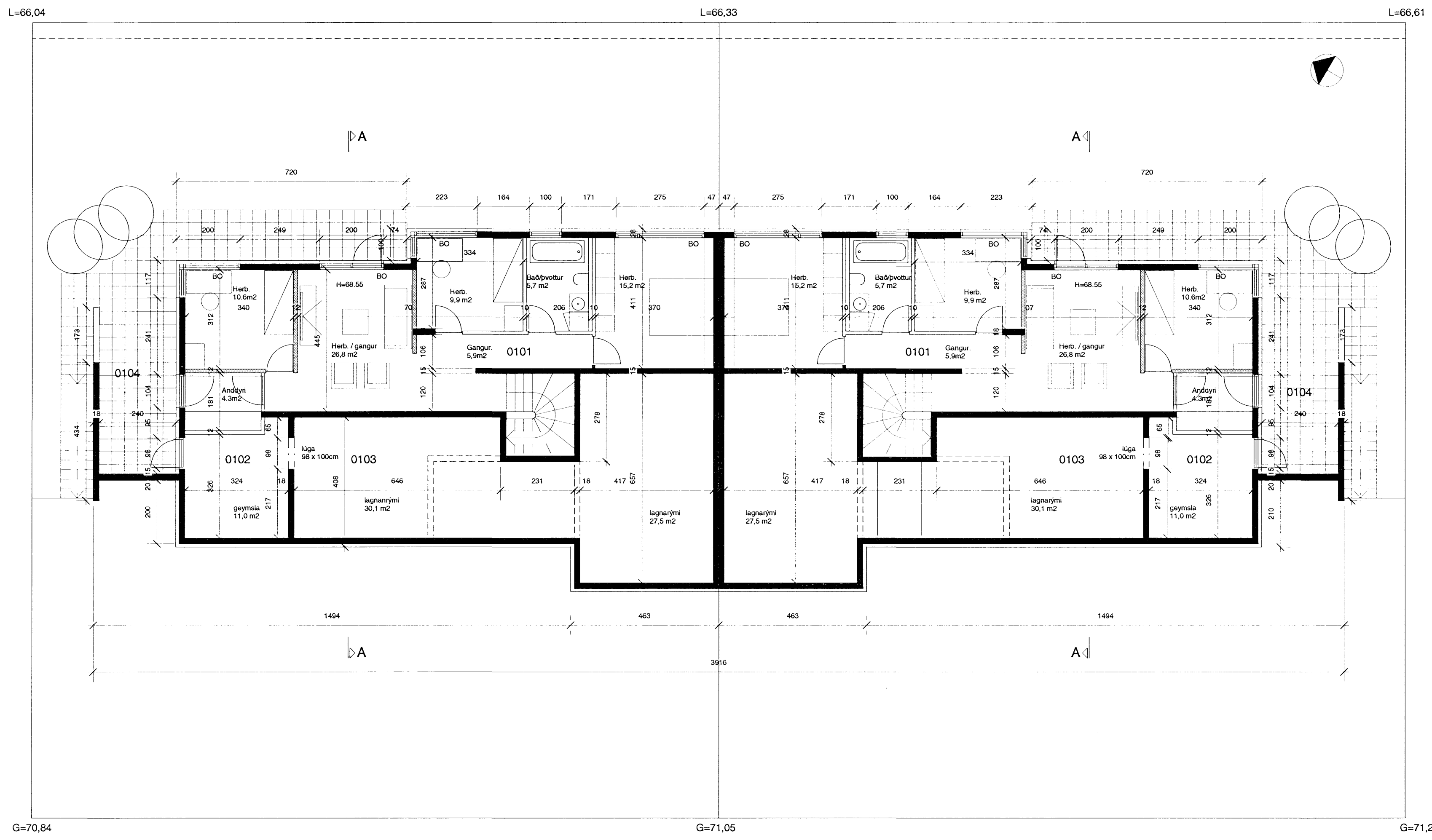
GRUNNMYND 1. HÆÐ
