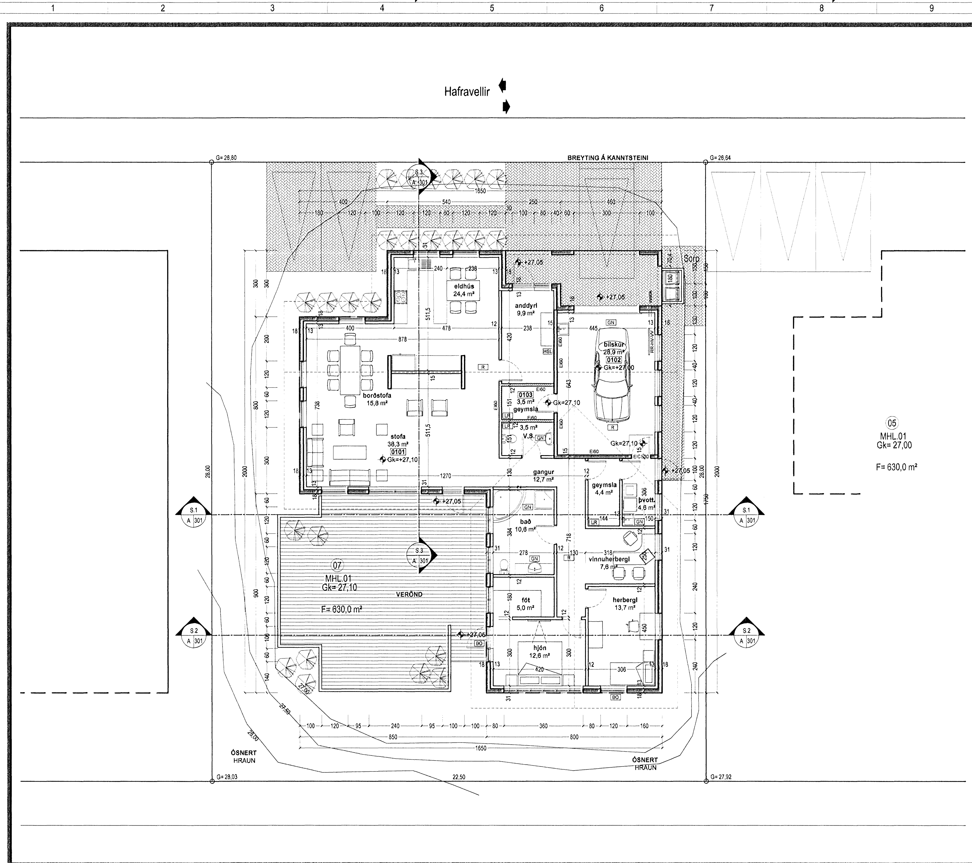
Grunnmynd 1:100
