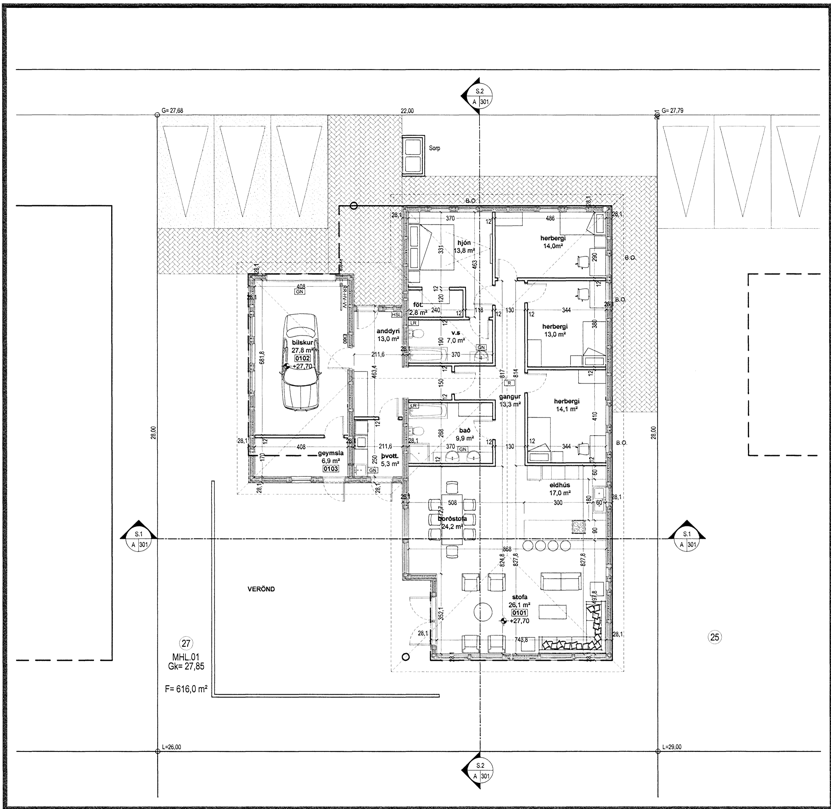
Grunnmynd 1:100
