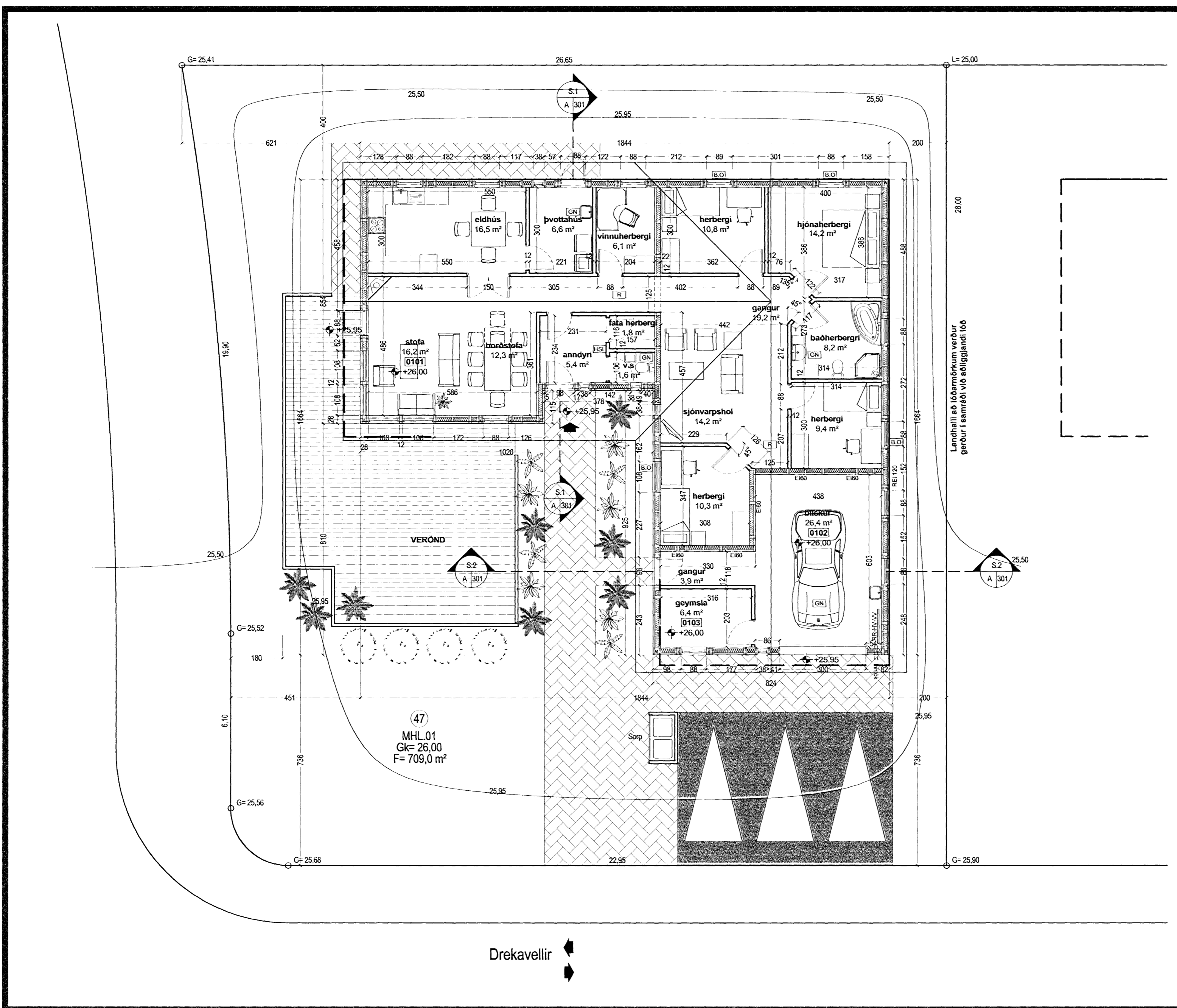
Grunnmynd 1:100
