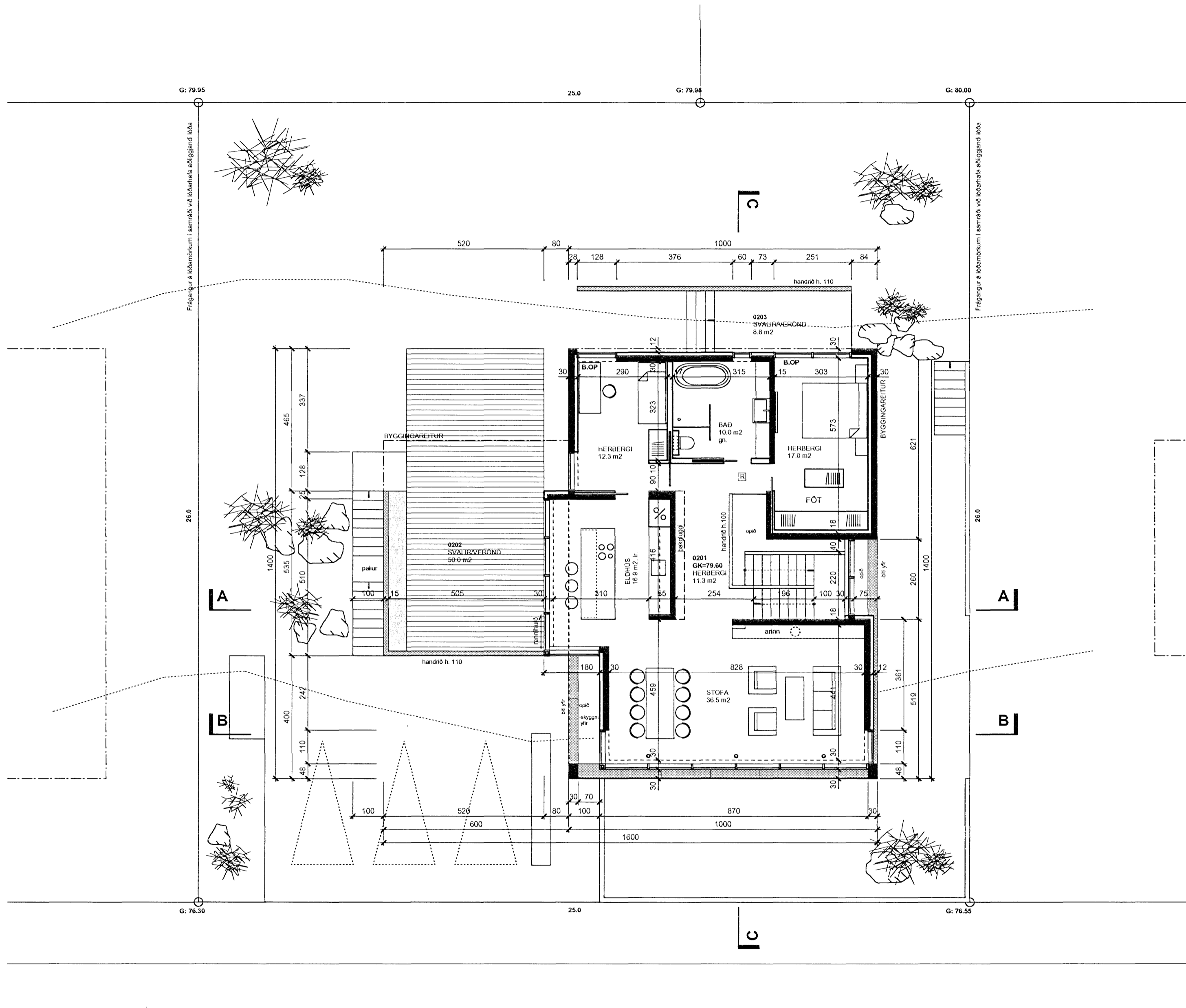
GRUNNMYND 2. HÆÐAR
