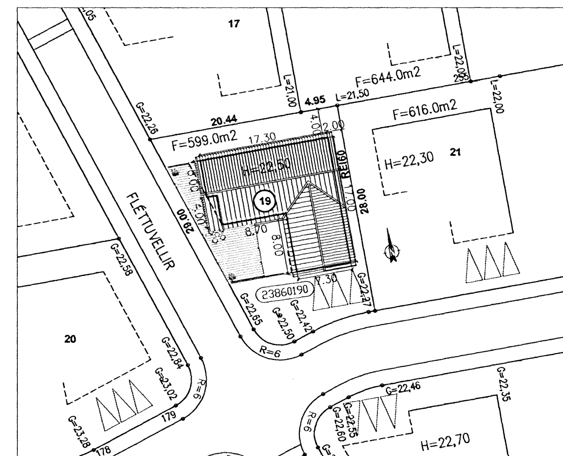
AFSTÖÐUMYND 1:500
