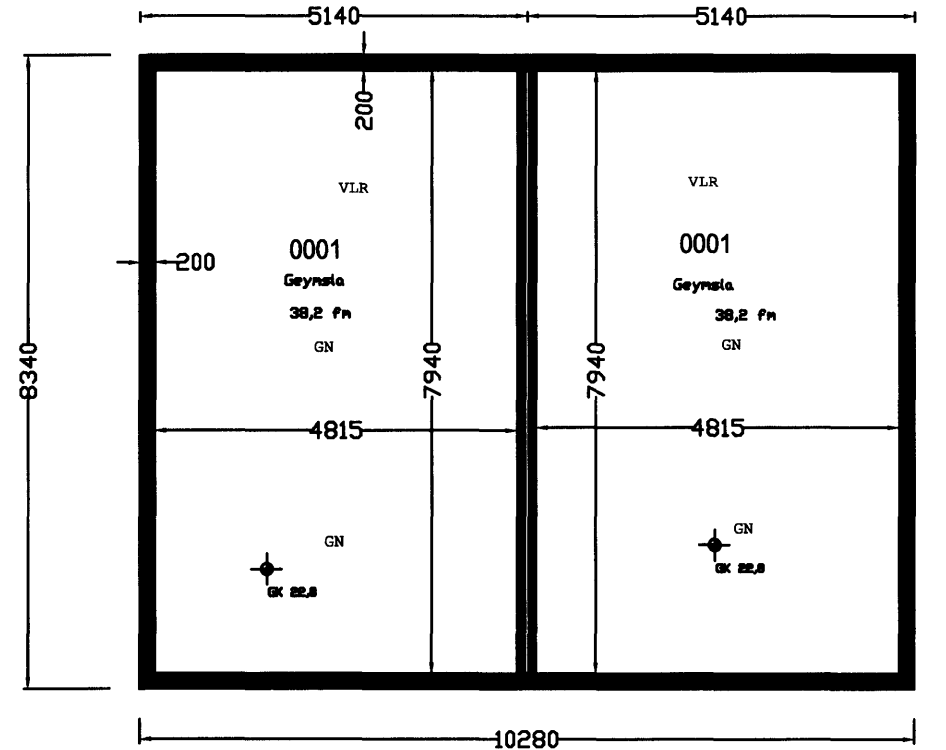
Grunnmynd kjallari / 0 hæð 0001 mkv: 1:100
