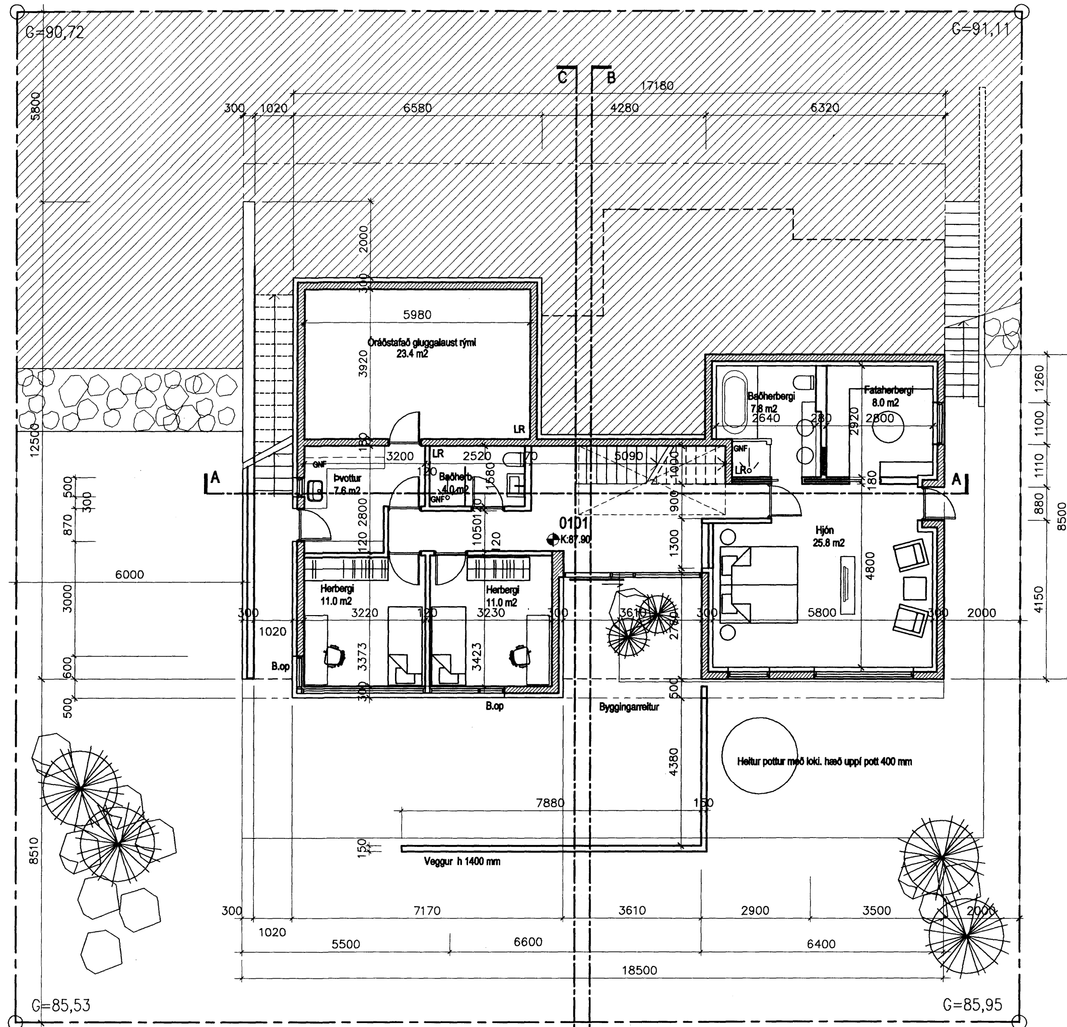
Grunnmynd 1. hæð
