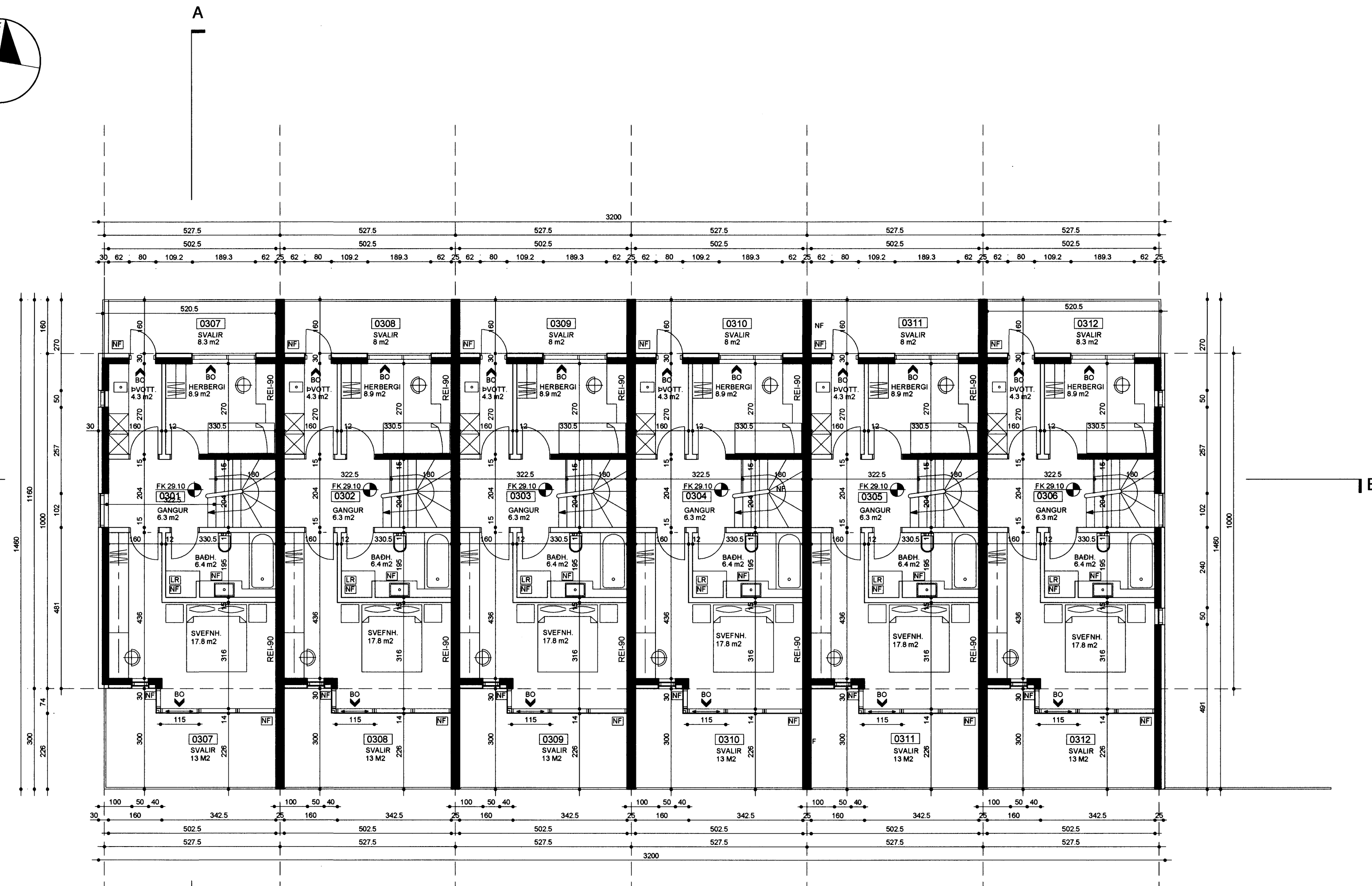
GRUNNMYND 3. HÆÐAR KVARDI 1:100
